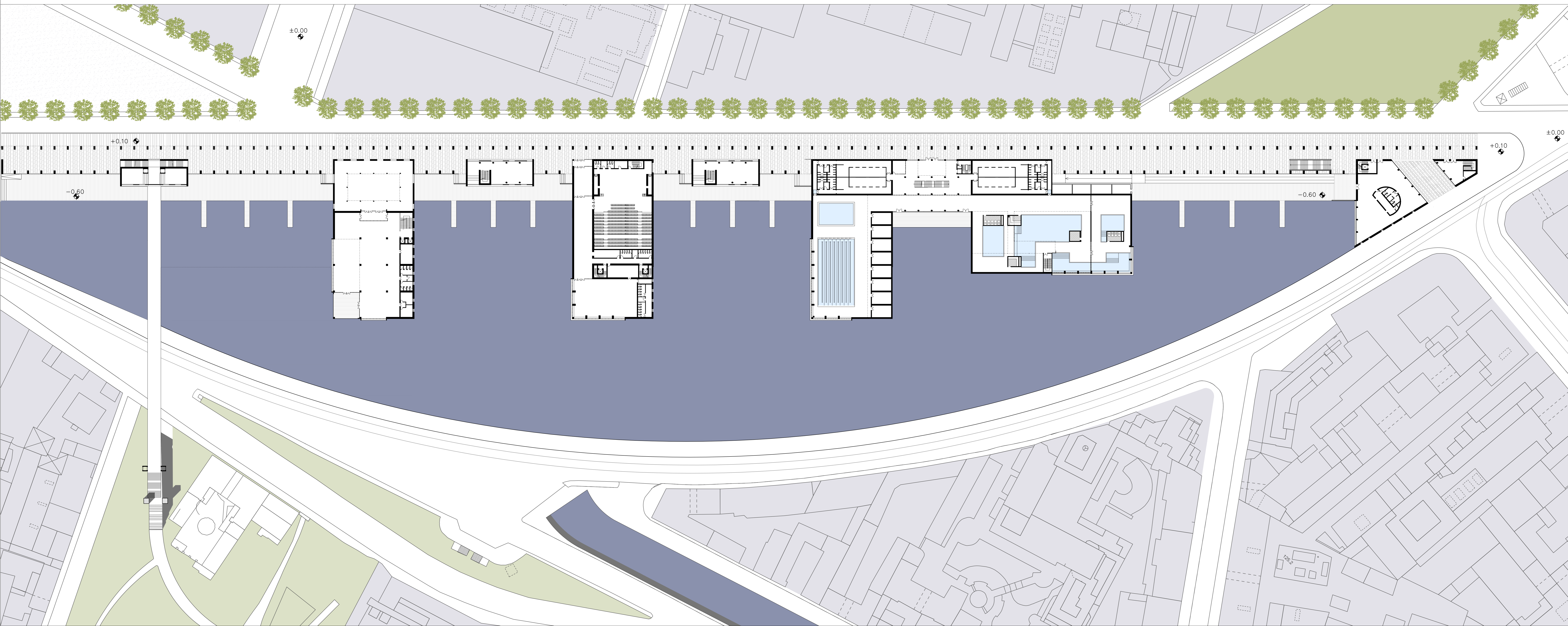
Planimetria generale_quota ±0.00 m_scala 1:500
