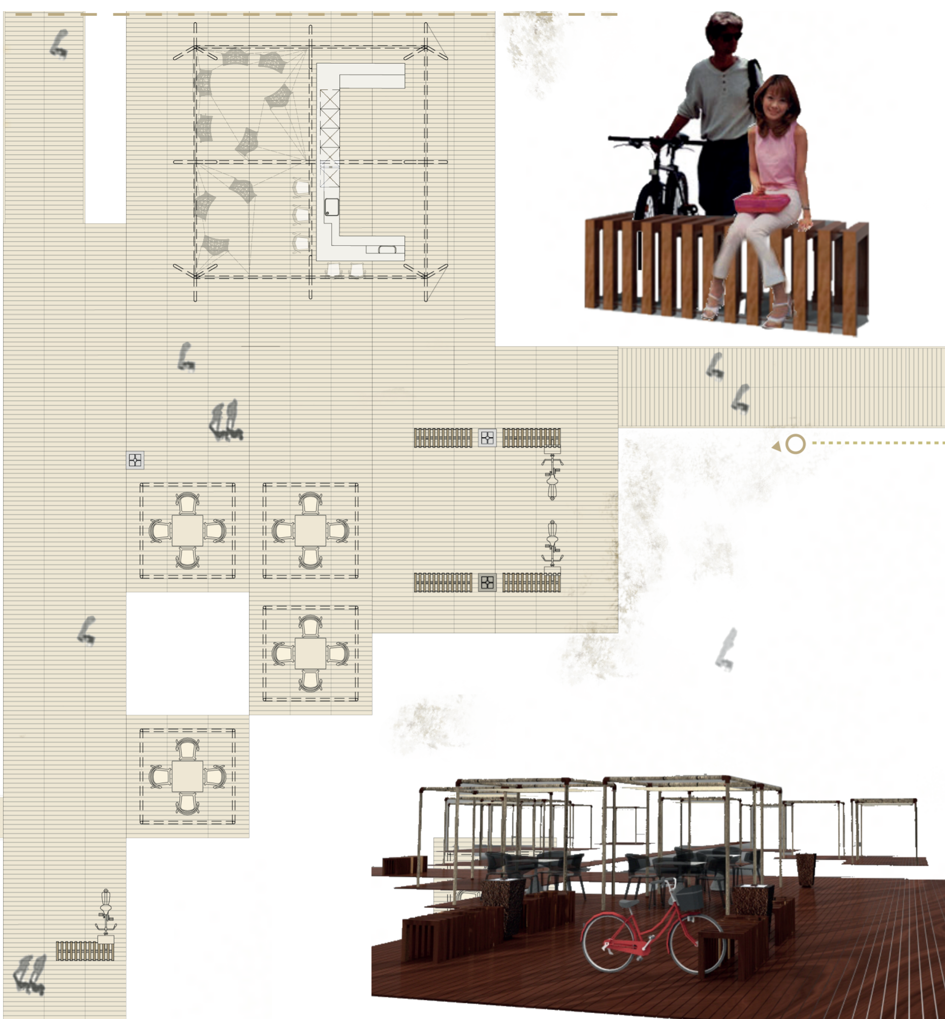
PIANTA AREA BAR scala 1:100
