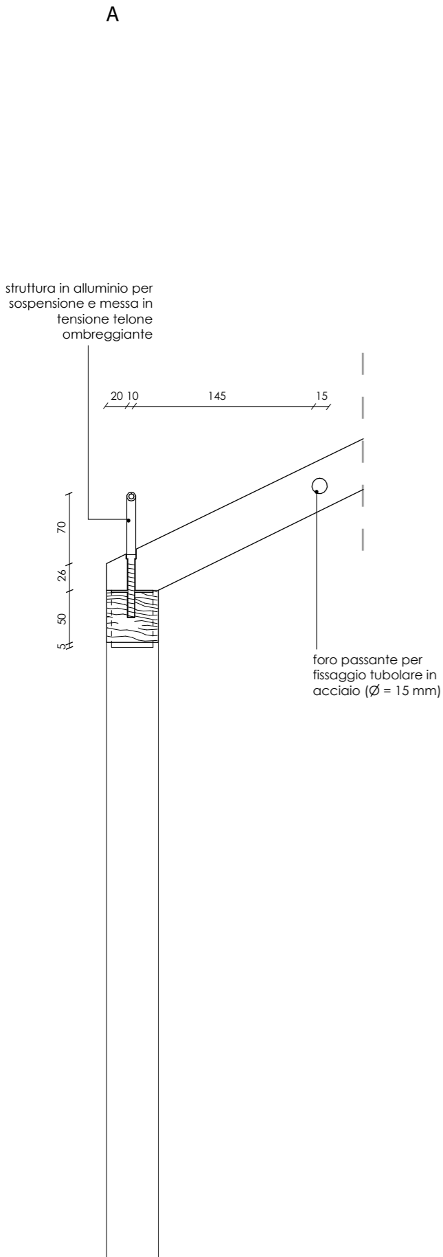
Dettagli nodi principali Scala 1:20
