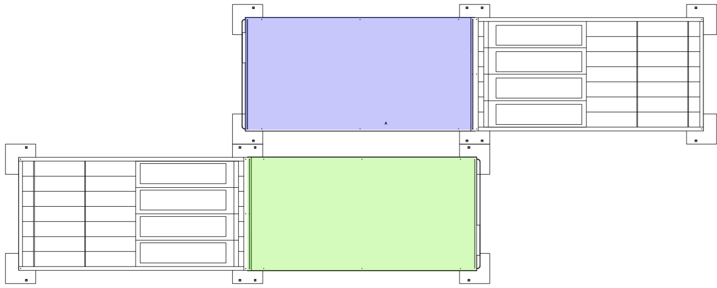
Tipologia aggregativa B Scala 1:50
