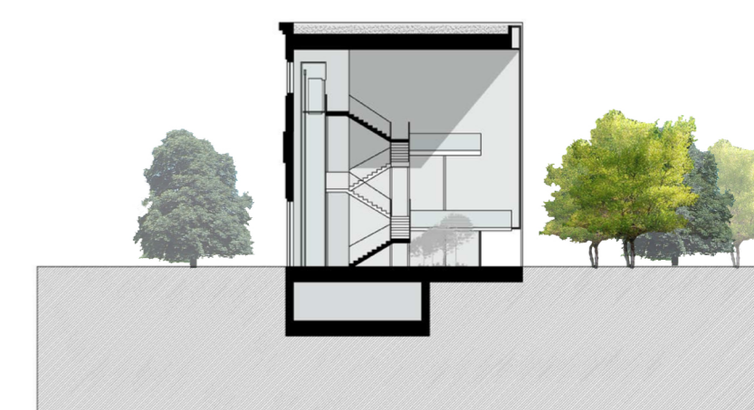
SEZIONE BB'
