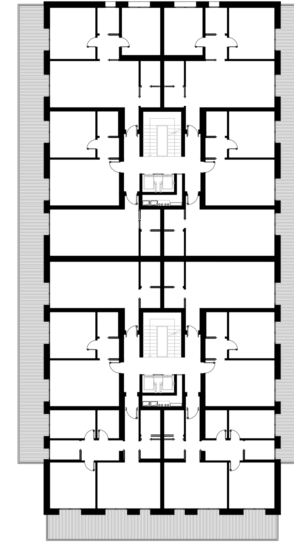
pianta tipo
