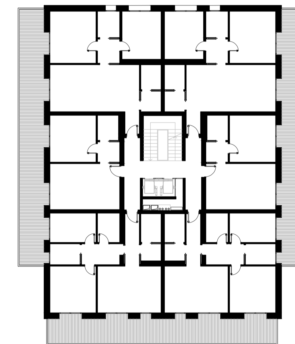
pianta tipo
