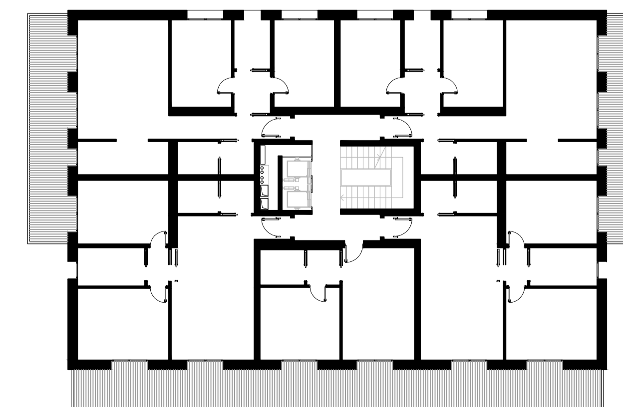
pianta tipo
