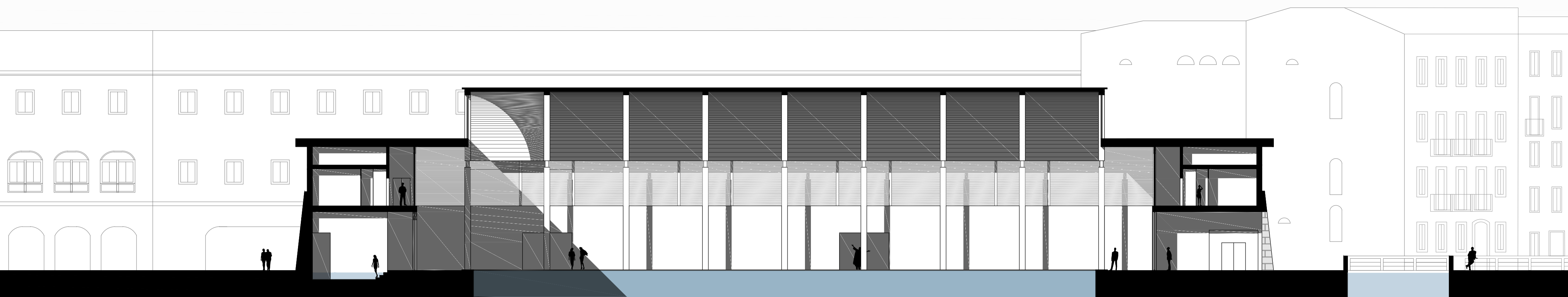
SEZIONE LONGITUDINALE DELLE TERME, SCALA 1:200
