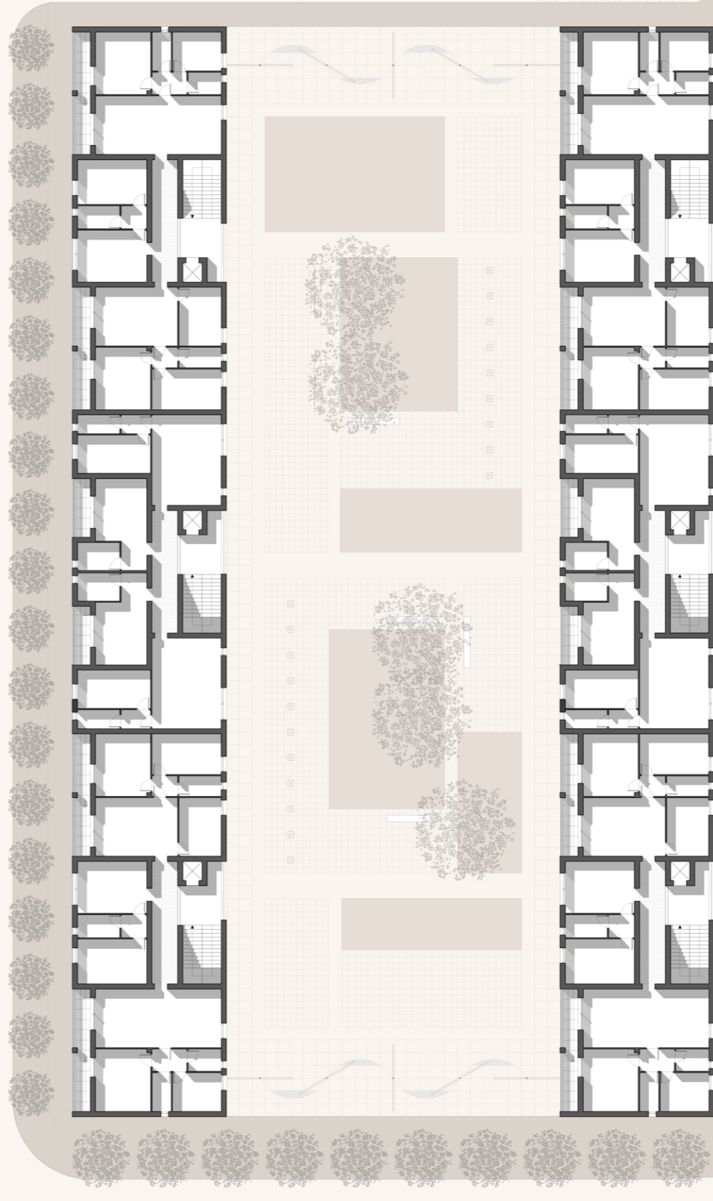
PIANO PRIMO
