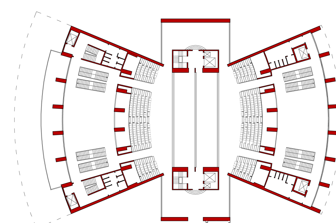
piano del primo foyer + 5,40 m
