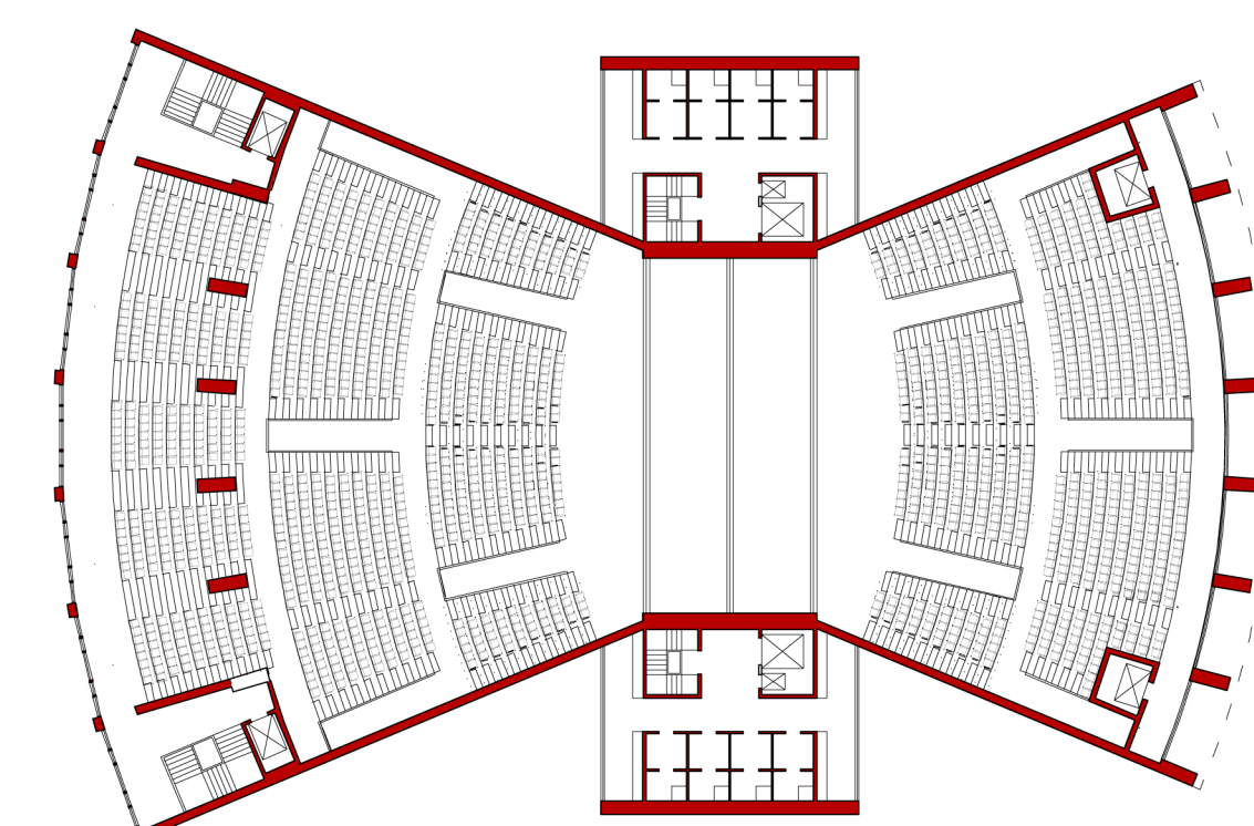
piano della galleria superiore + 15,60 m
