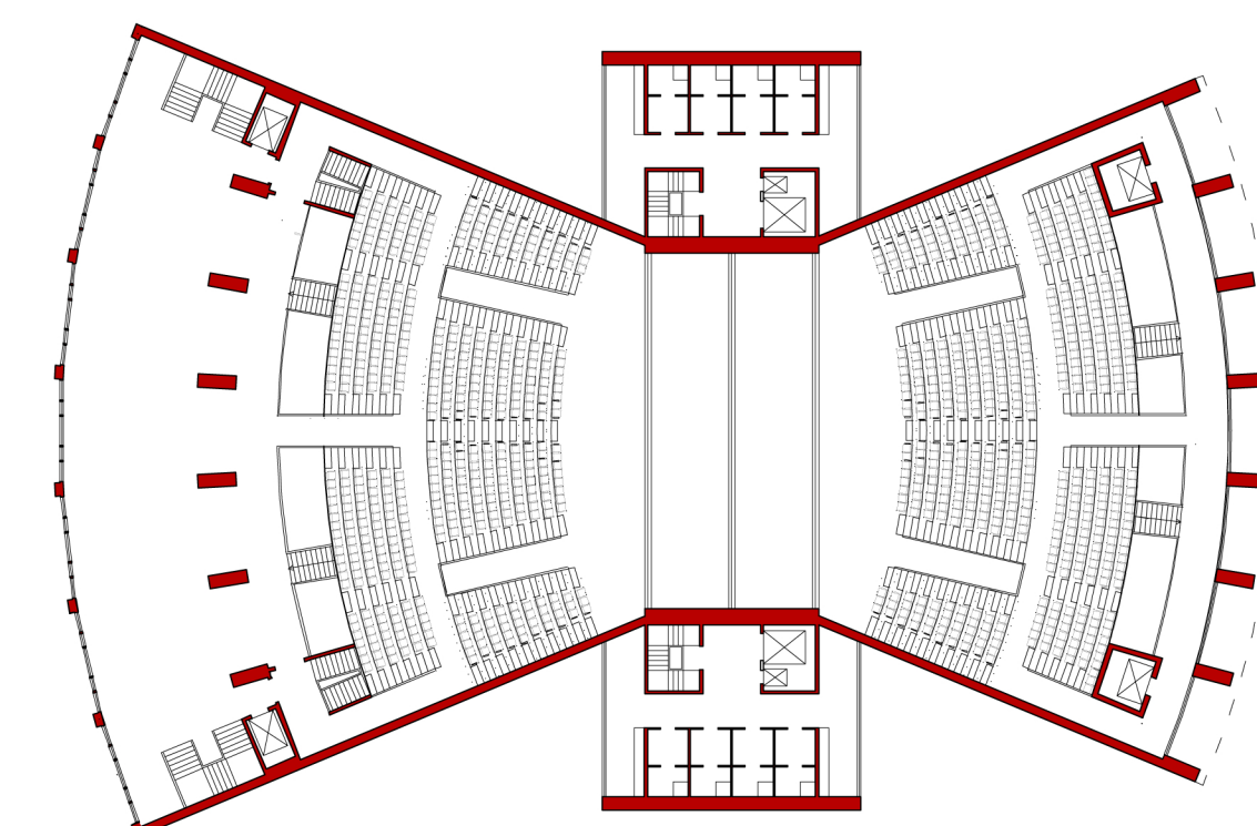
piano del secondo foyer + 8,80 m
