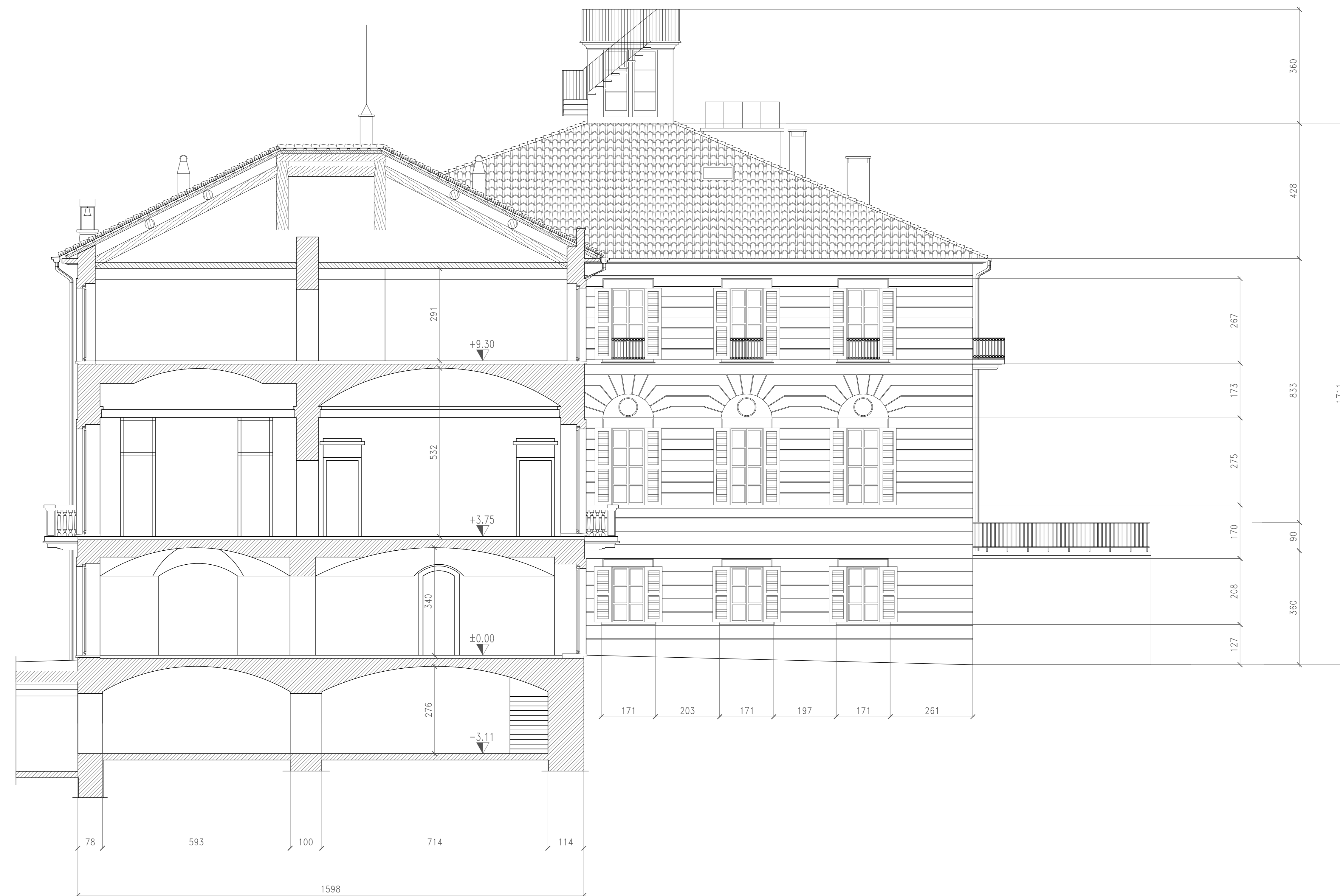
SEZIONE D-D'
