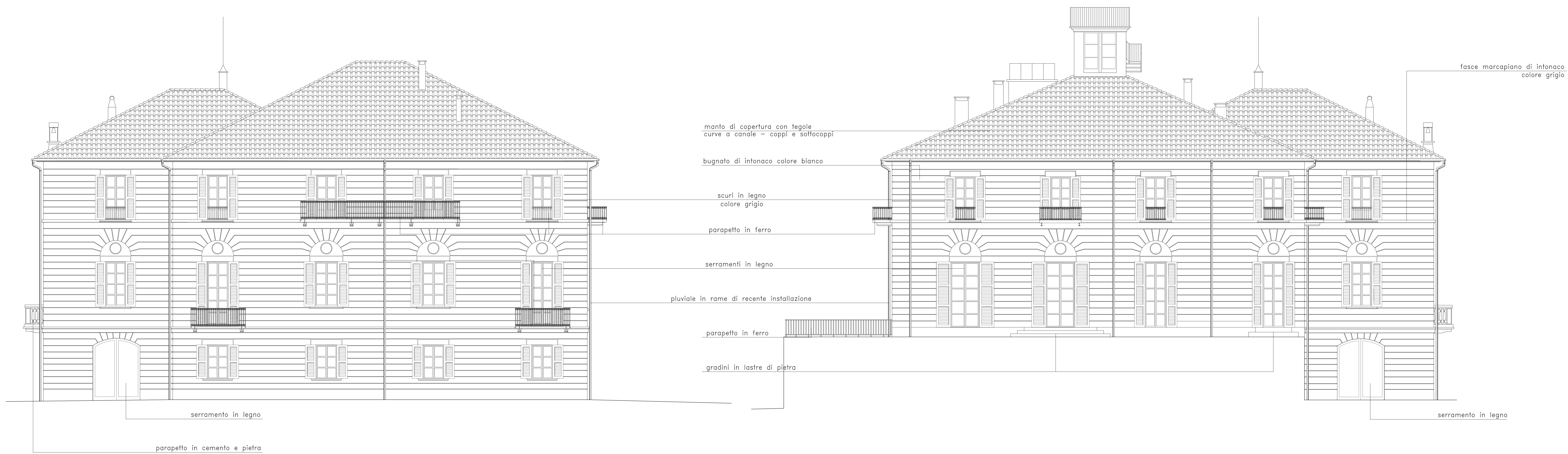
PROSPETTO EST
