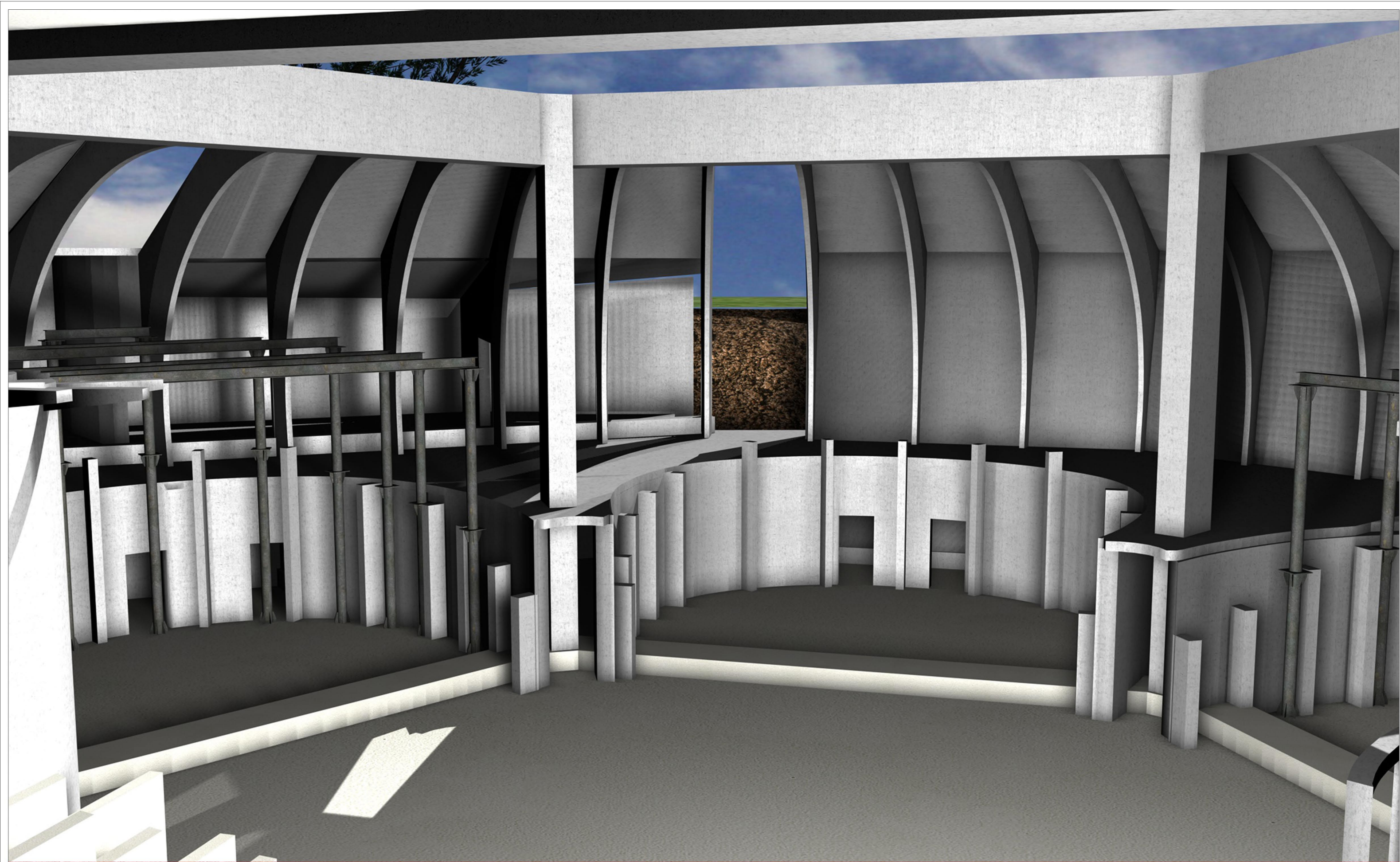
FASE 17: Getto della costolatura del corridoio e getto del suo solaio.
