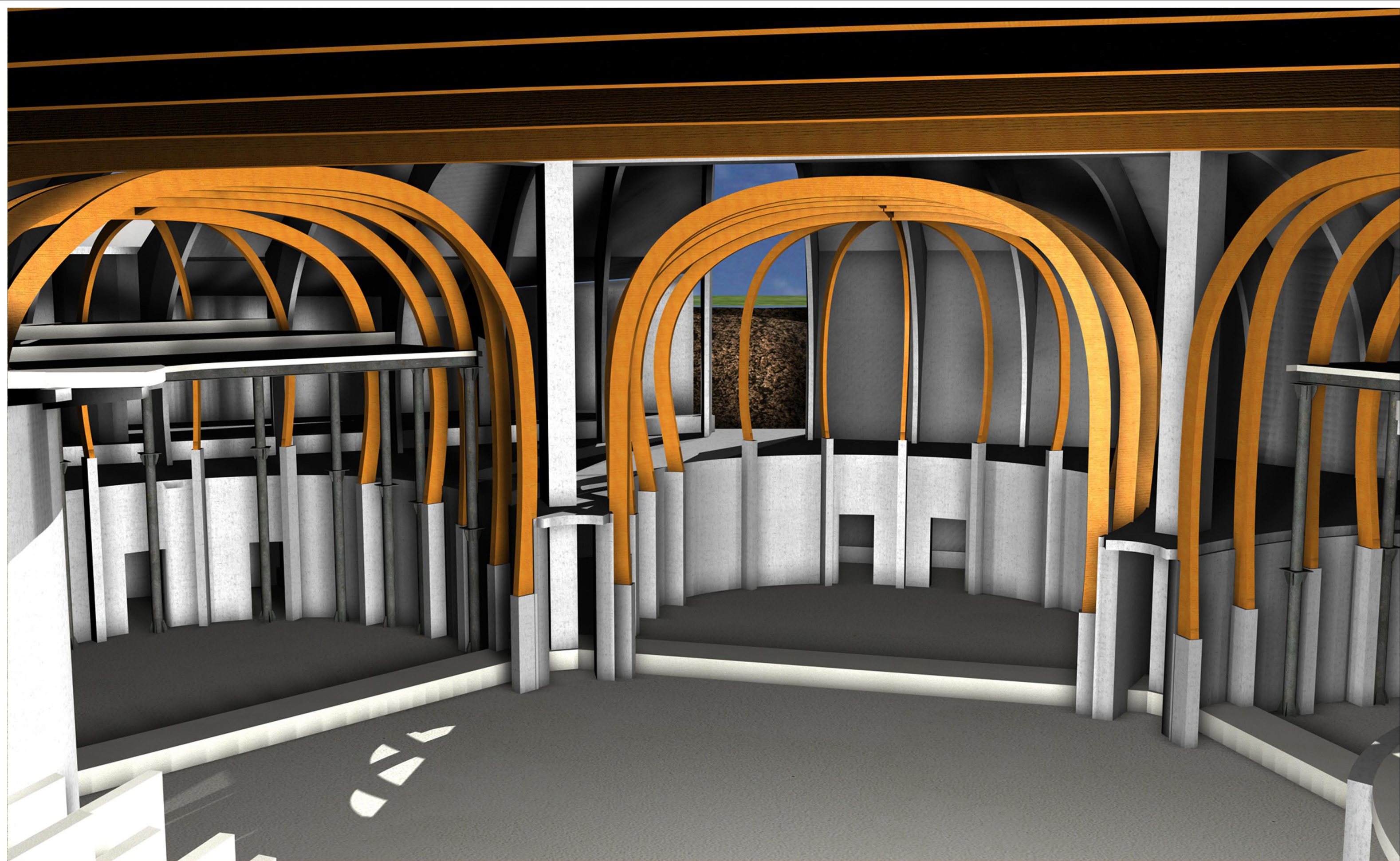
FASE 19: Getto della soletta della galleria sopra le HEA (muniti di pioli Nelson).
