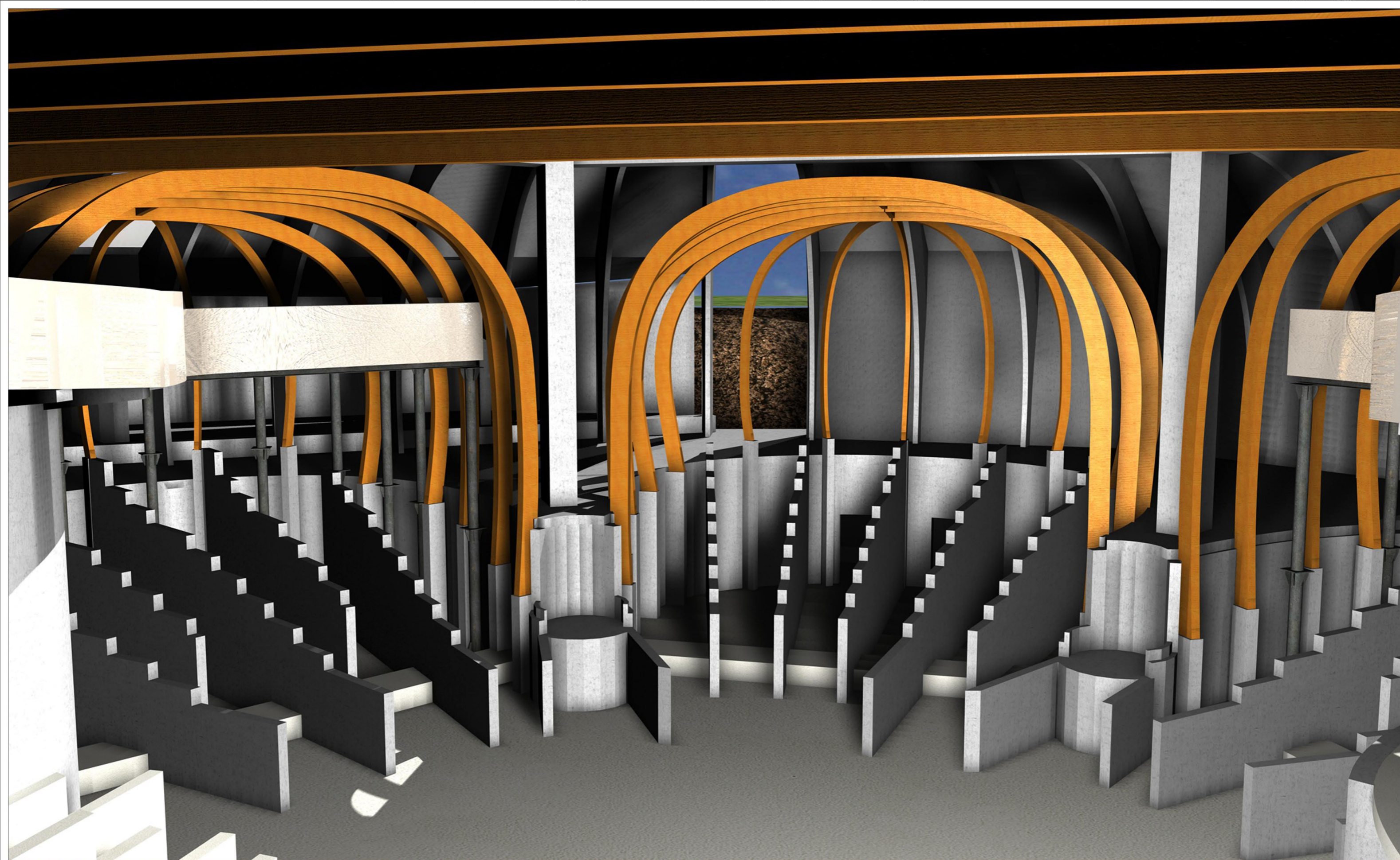
FASE 21: Getto delle costolature dei lobi est, nord e ovest.
