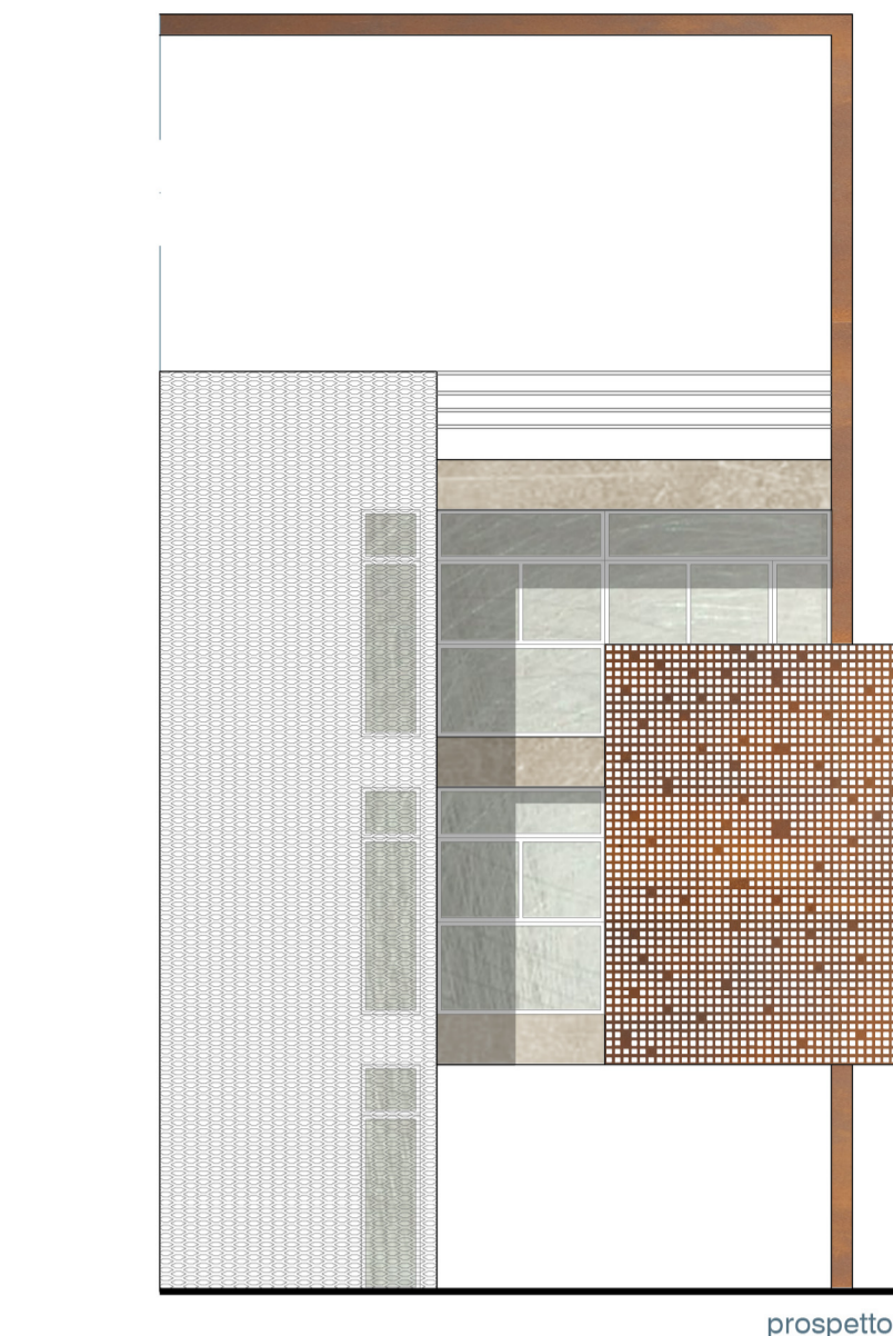
prospetto est
