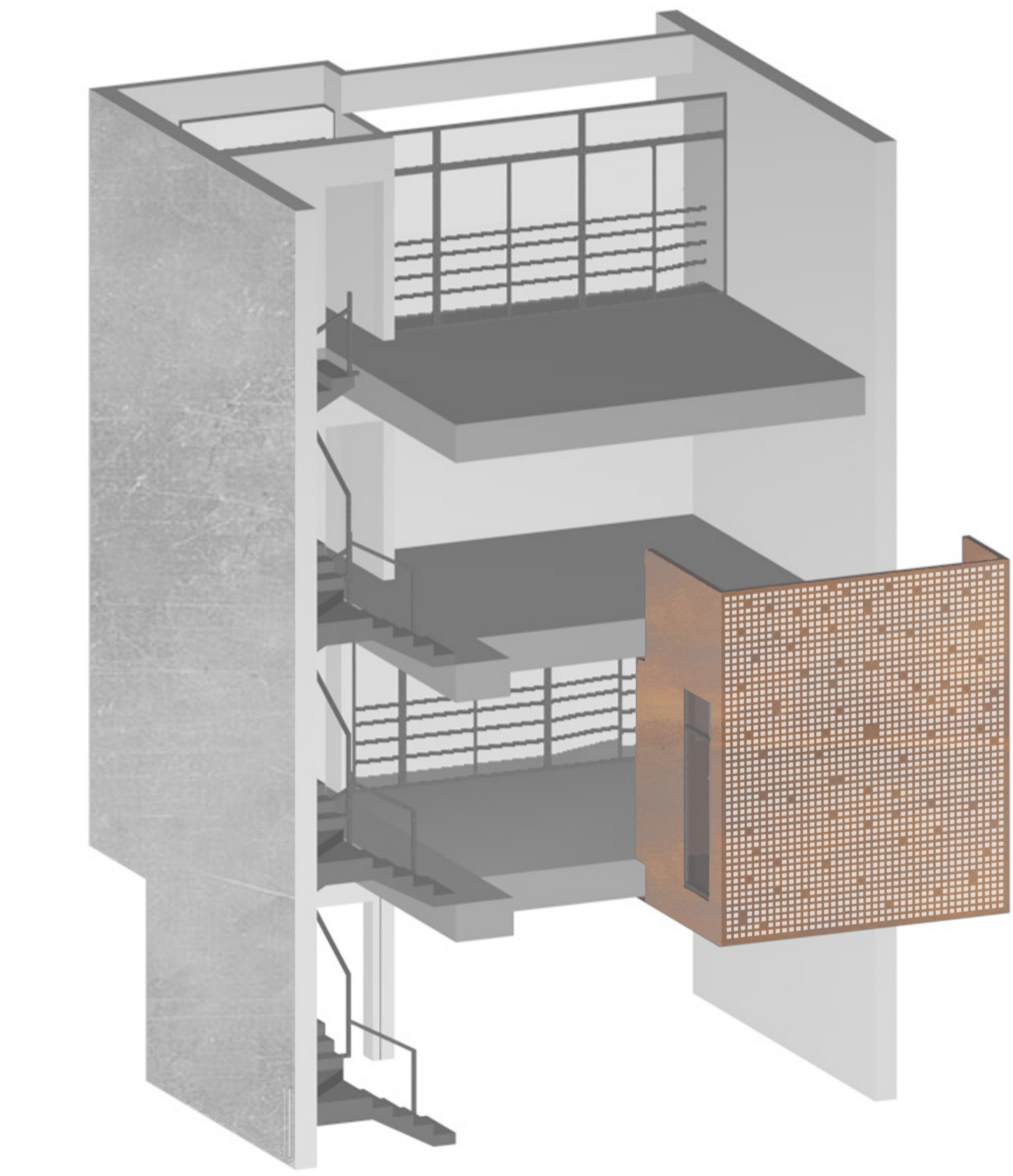
spaccato assonometrico
