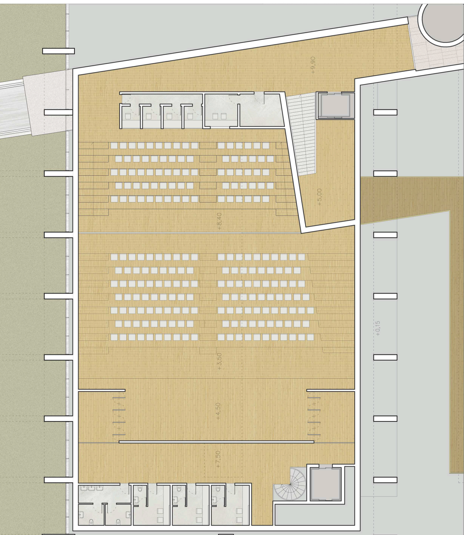
PIANTA AUDITORIUM +990
