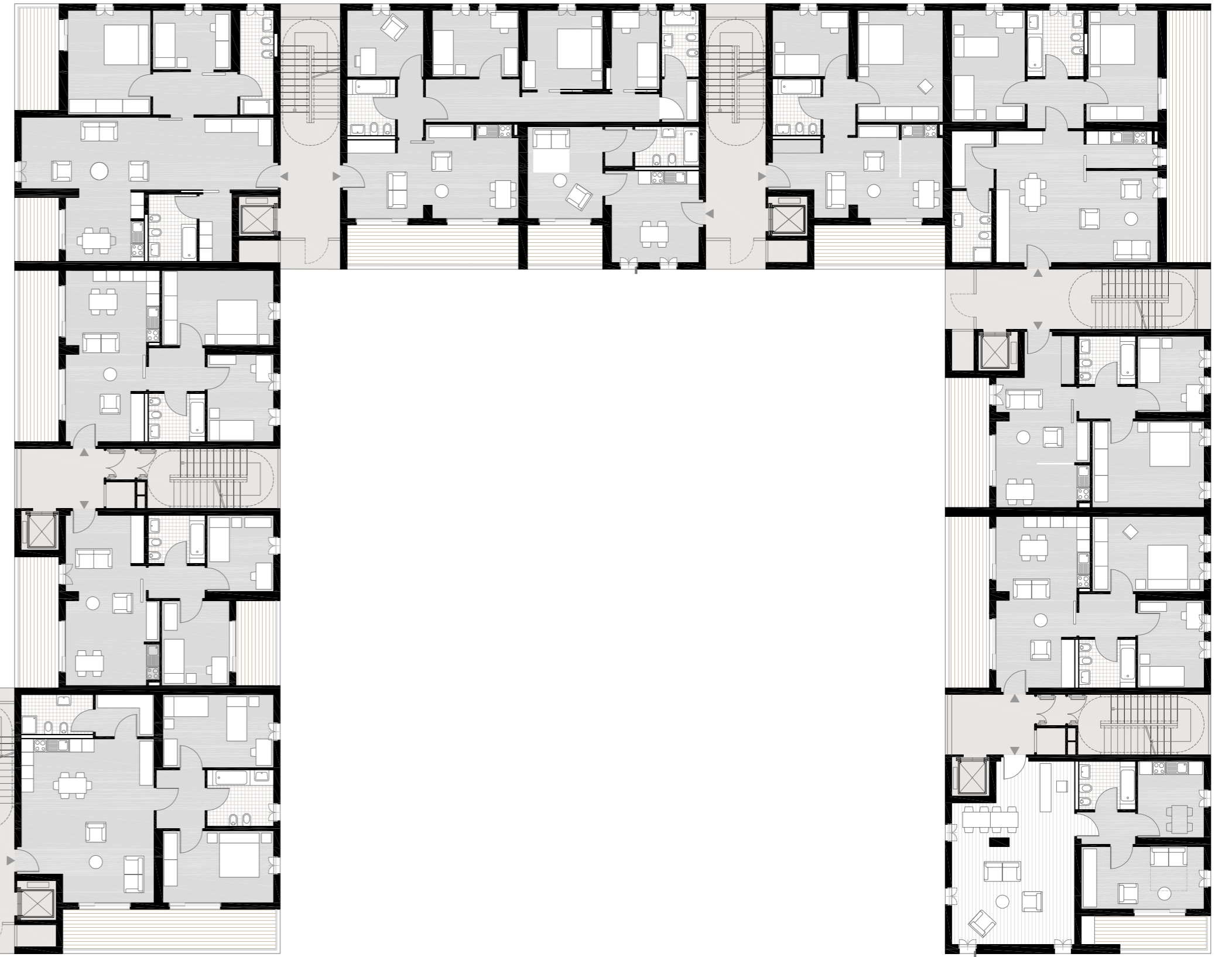
Torre 4, piani successivi
