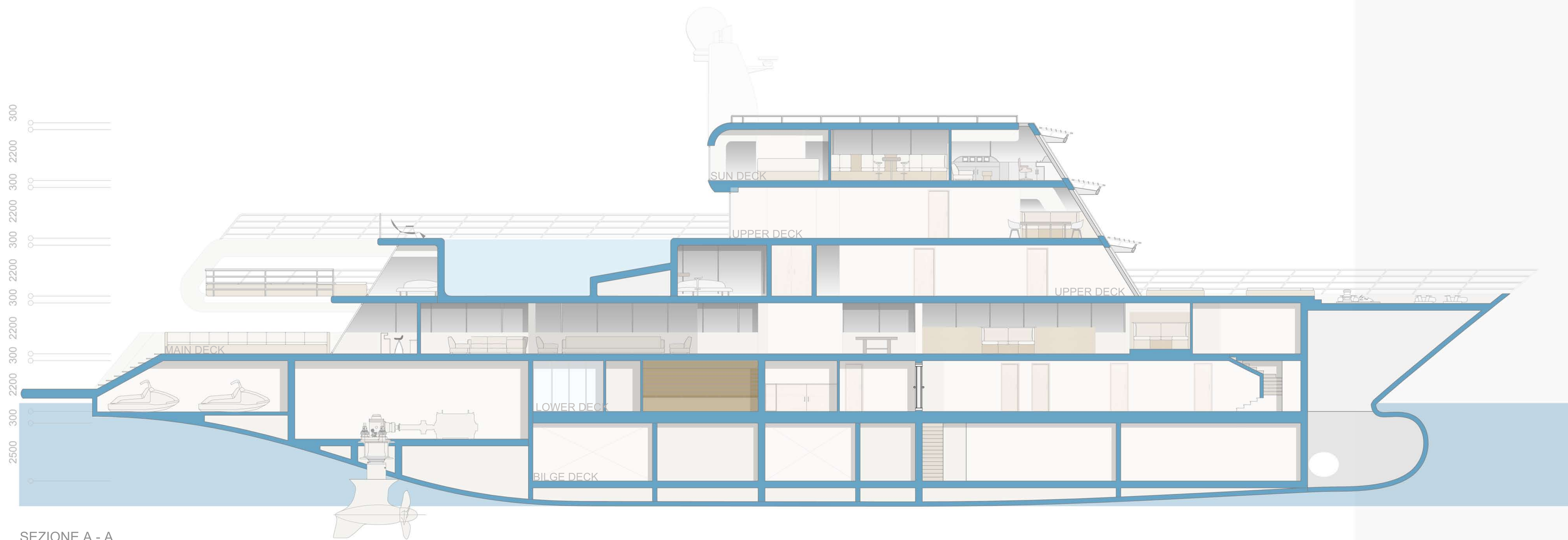
SEZIONE A - A
