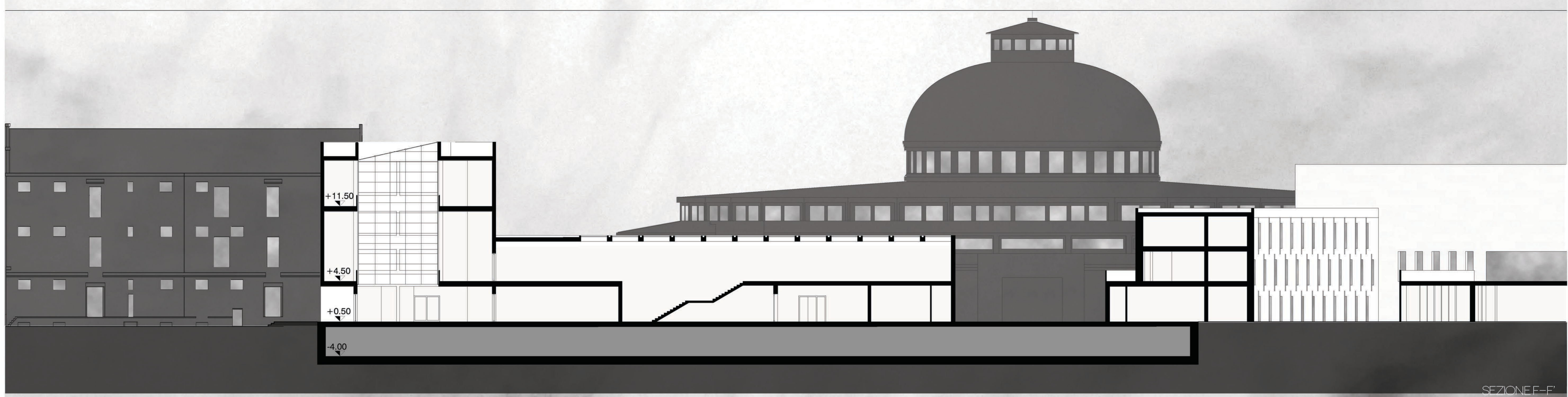
SEZIONE E-F
