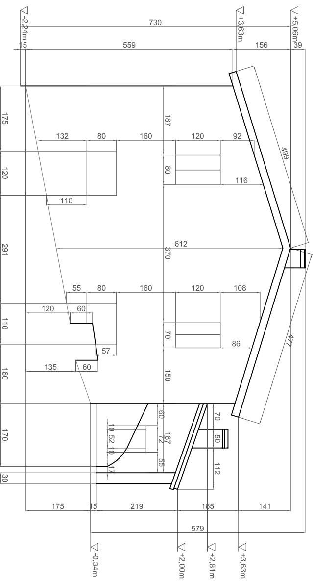
Prospetto Sud
