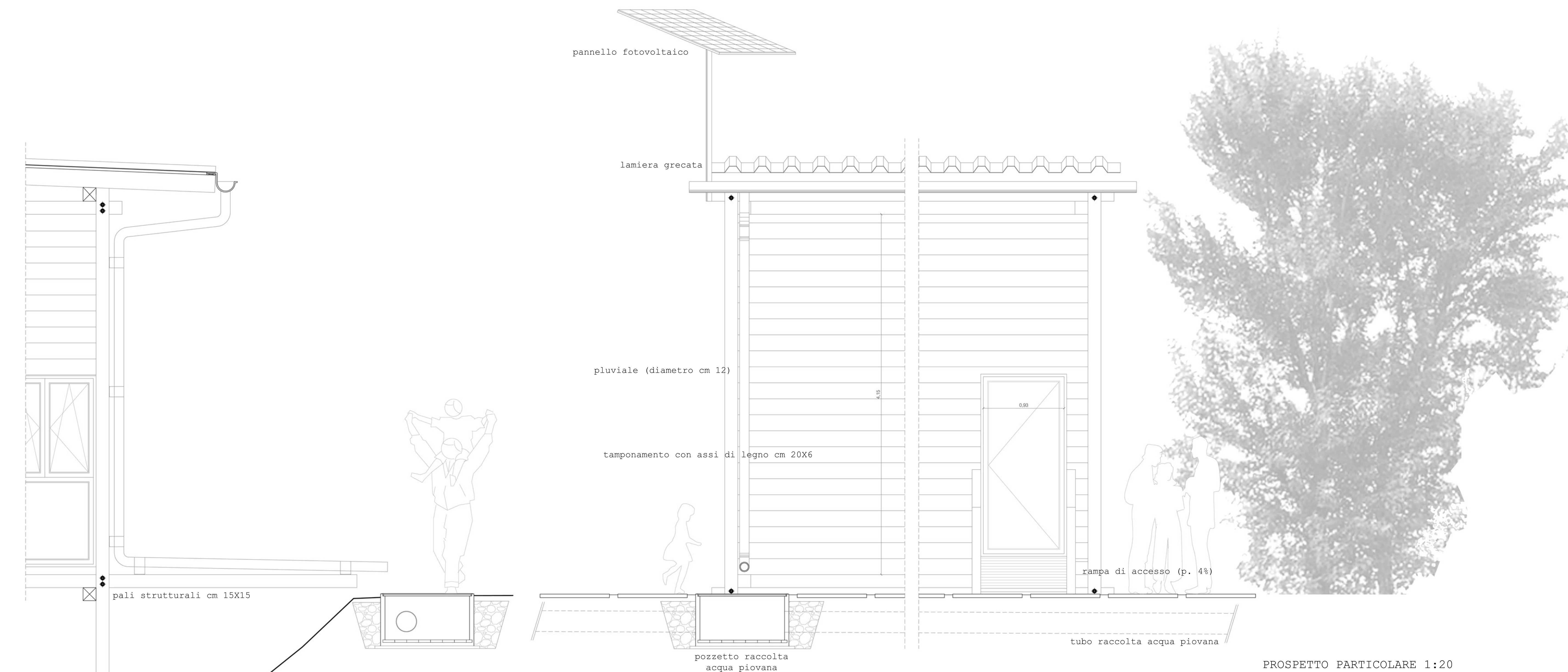
PROSPETTO PARTICOLARE 1:20
