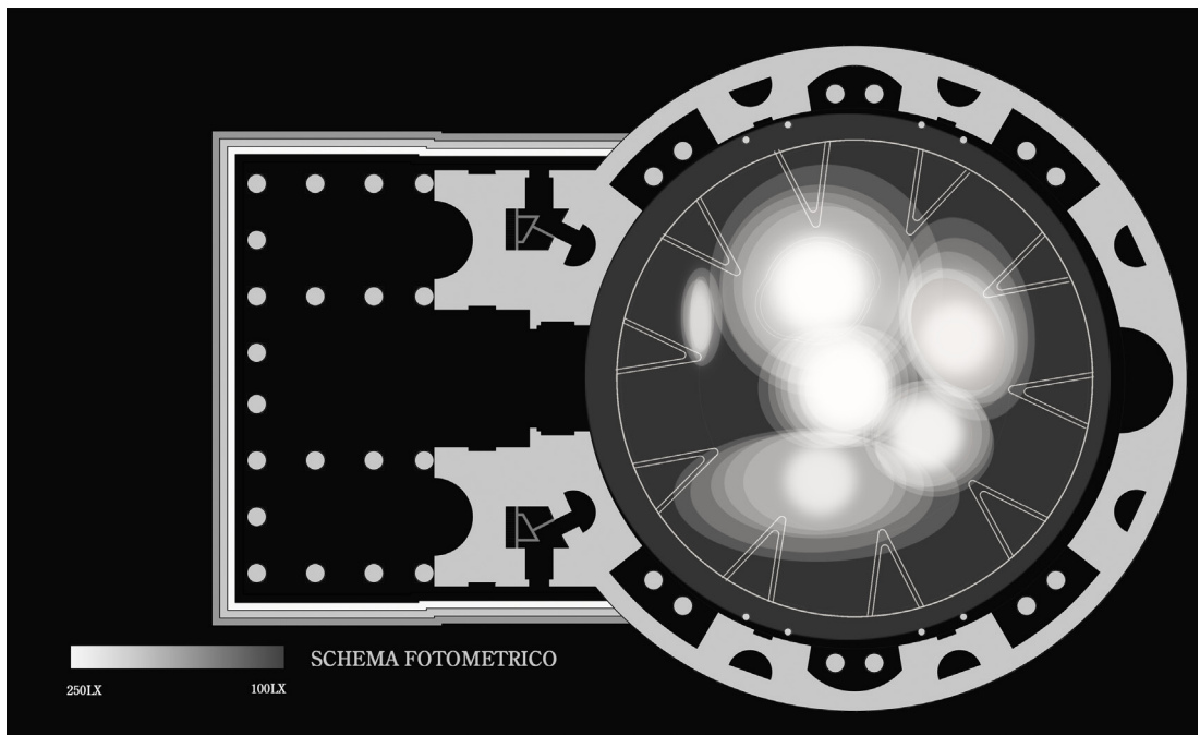
Fig.74 Schema fotometrico
