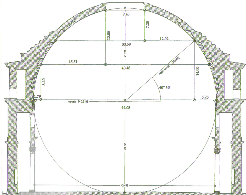
Fig.58 la geometria della cupola e del cilindro
