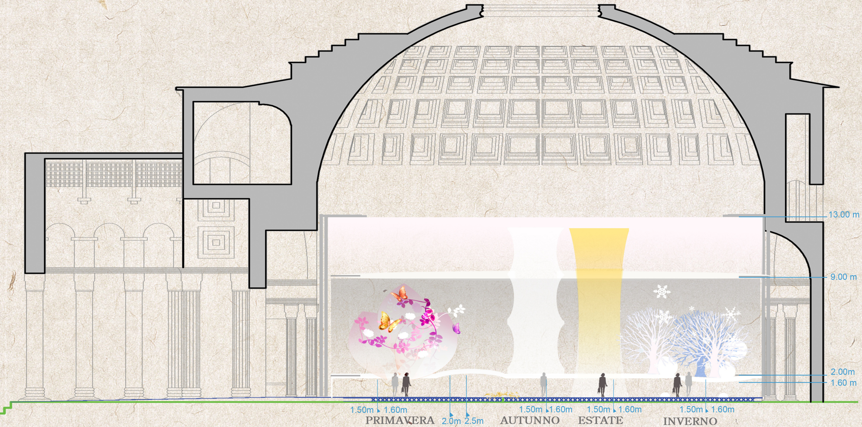
Fig.76 Sezione di progetto
