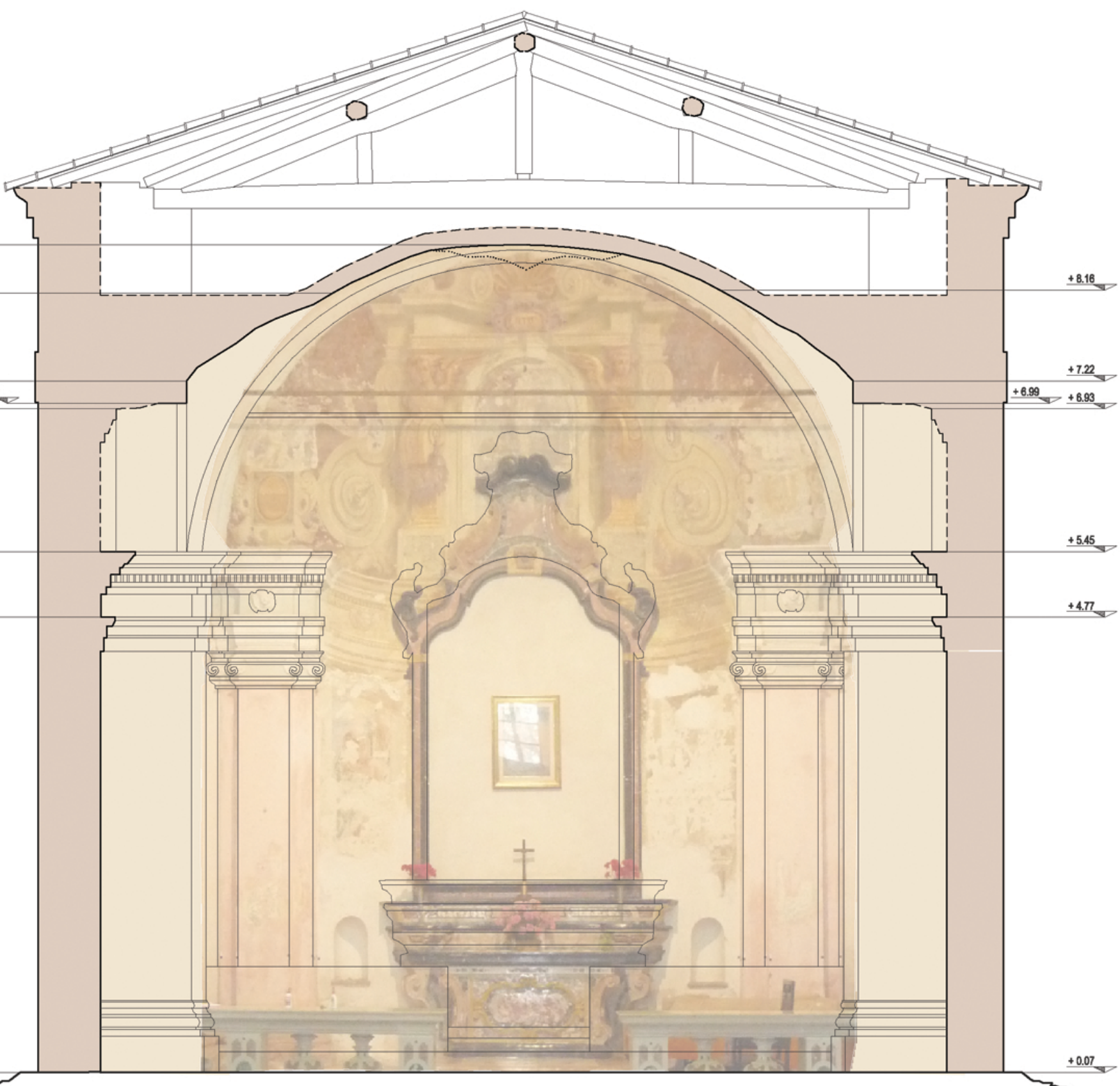
Sezione CC'
