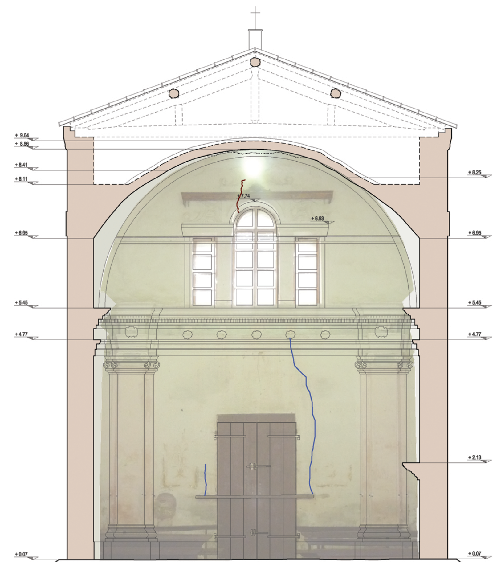
Sezione DD'
