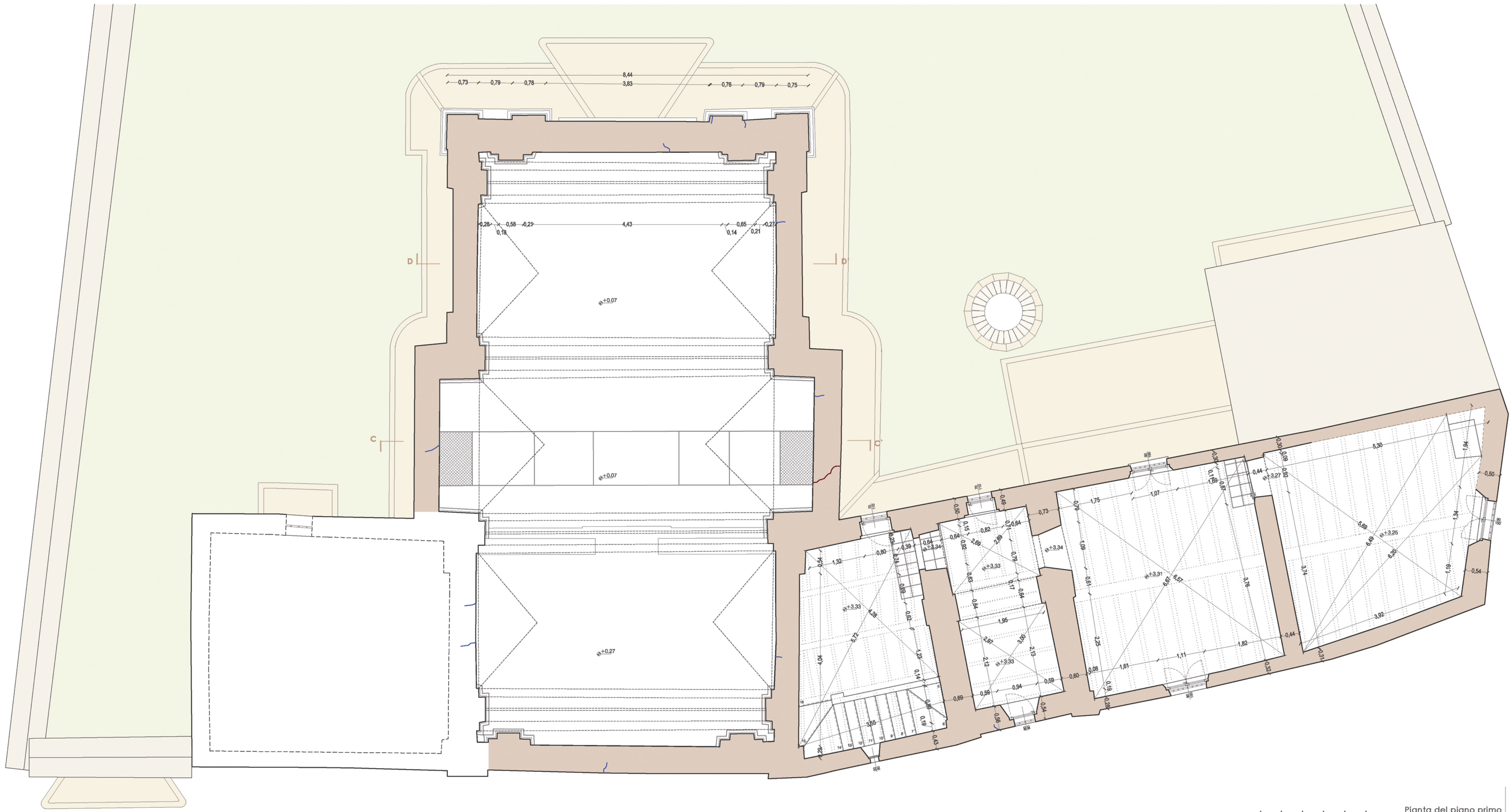
Pianta del piano primo
