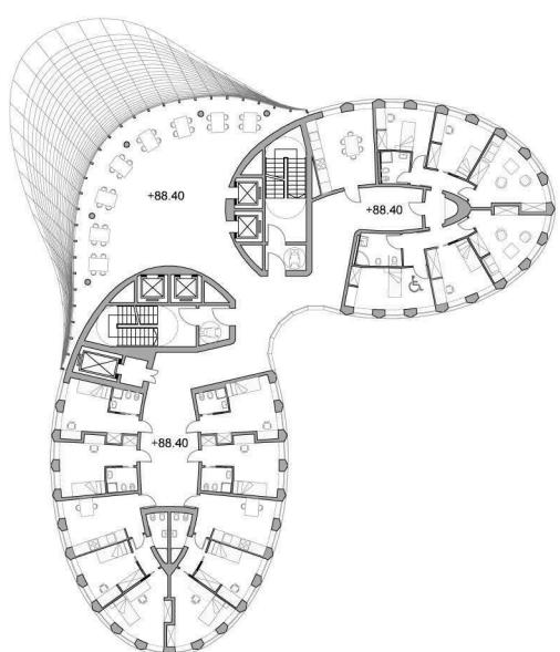
PIANTA PIANO TIPO PROFESSORI
