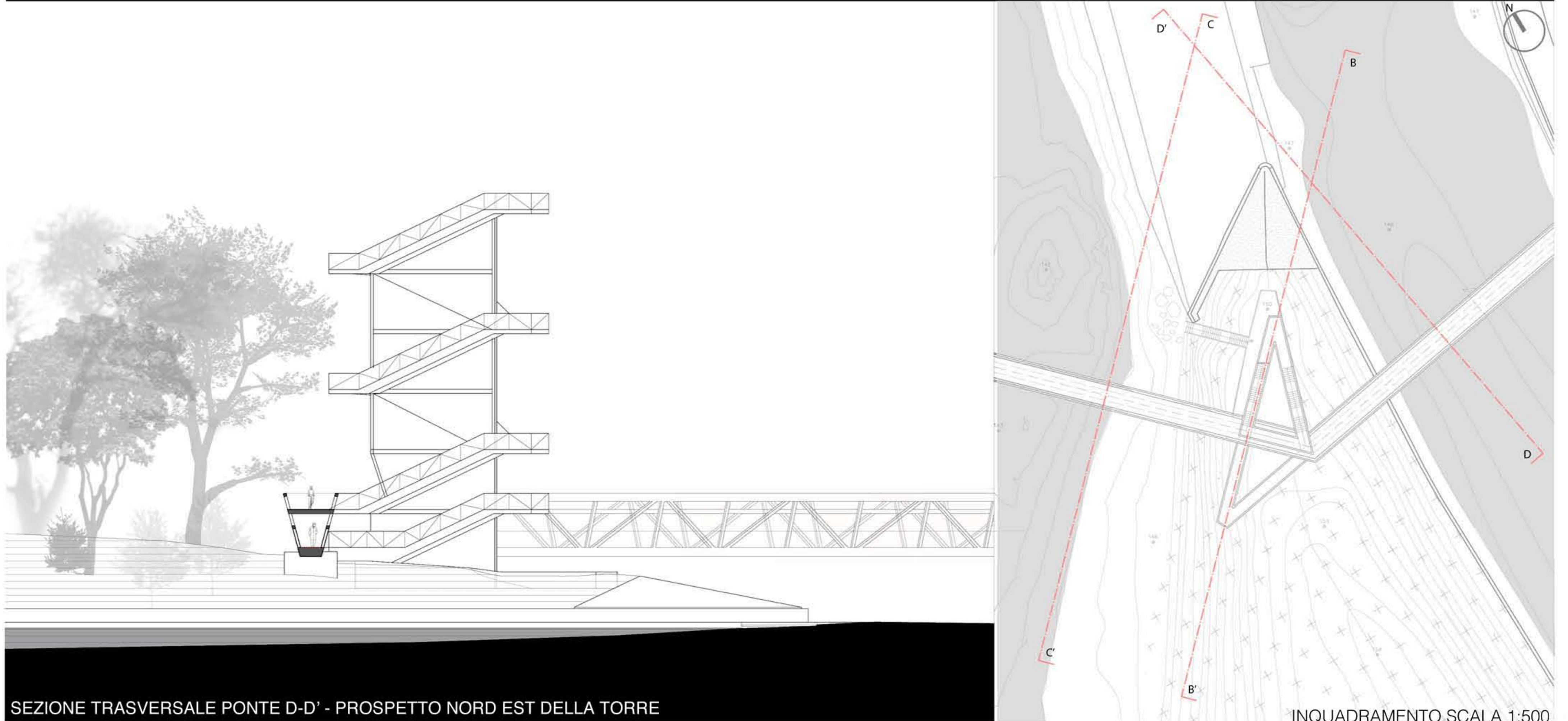
SEZIONE TRASVERSALE PONTE C-C' - PROSPETTO OVEST DELLA TORRE
