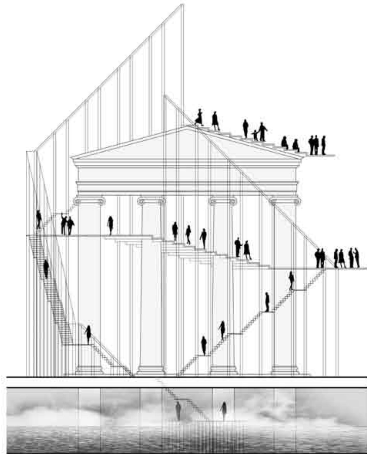
prospetto nord scala 1 : 100
