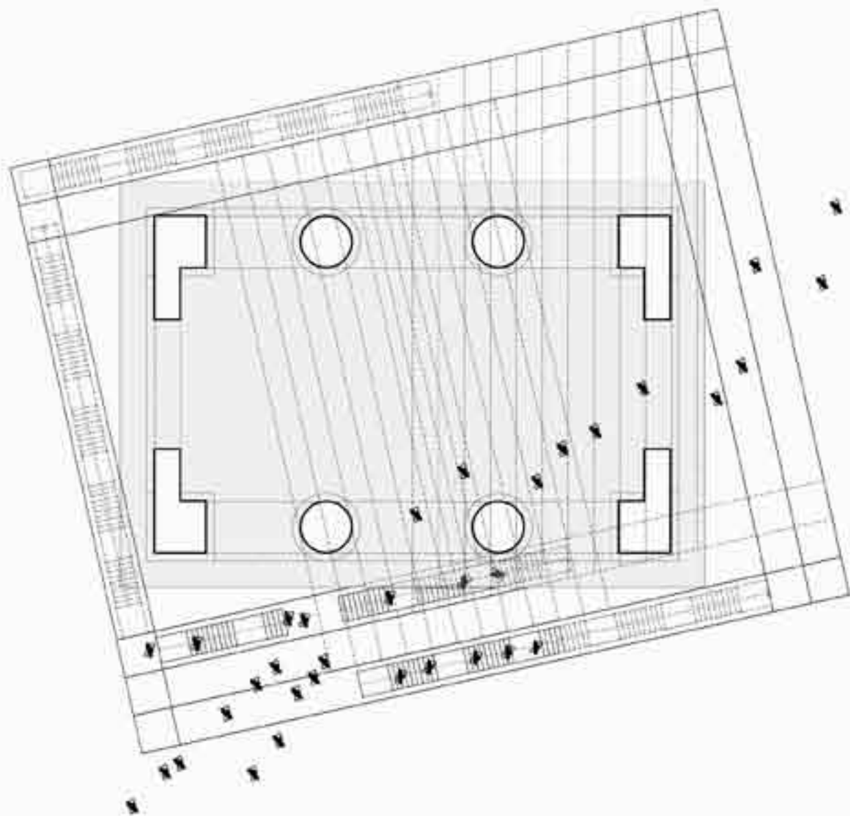
pianta livello \pm 0.00 m scala 1 : 100
