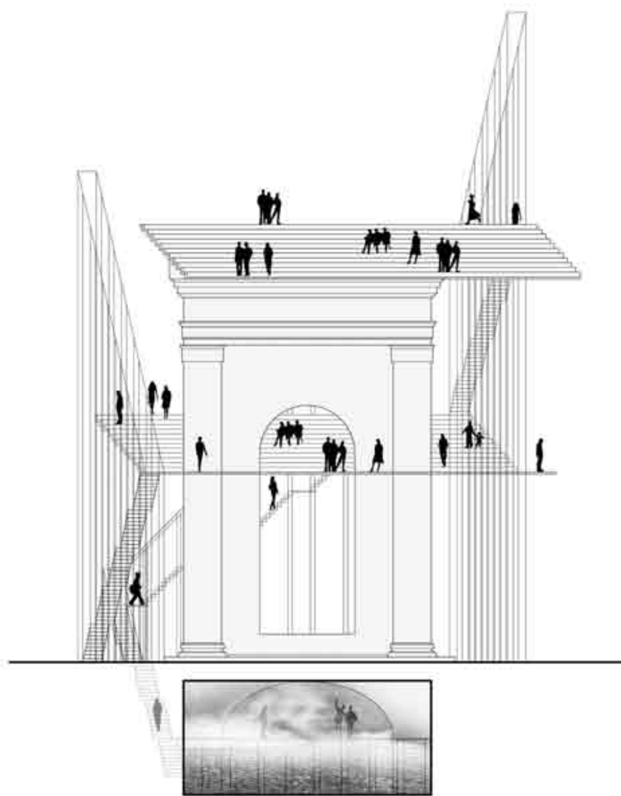
prospetto ovest scala 1 : 100
