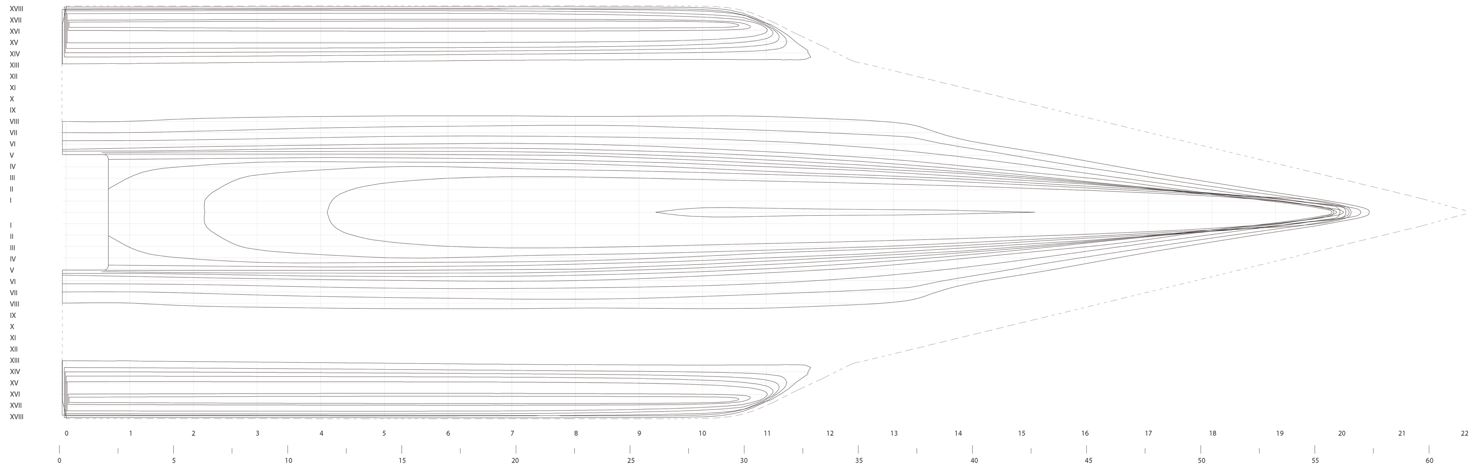
Piano delle linee d'acqua_pianta
