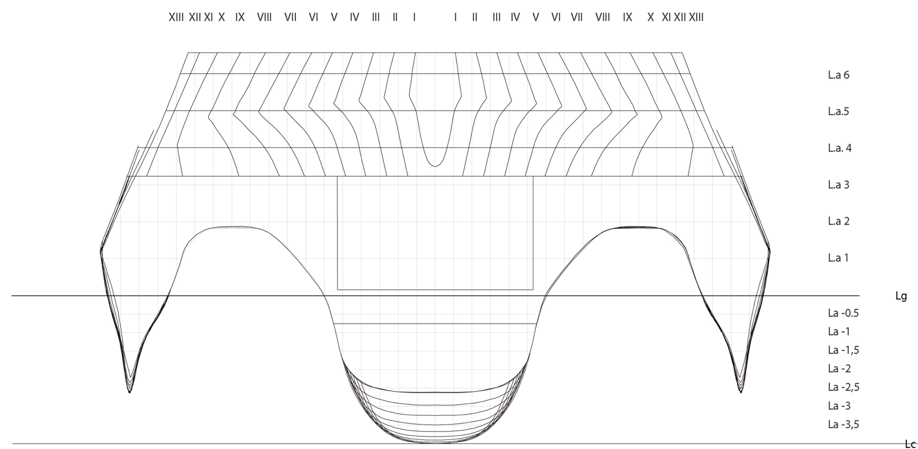
Piano delle ordinate_sezioni verticali
