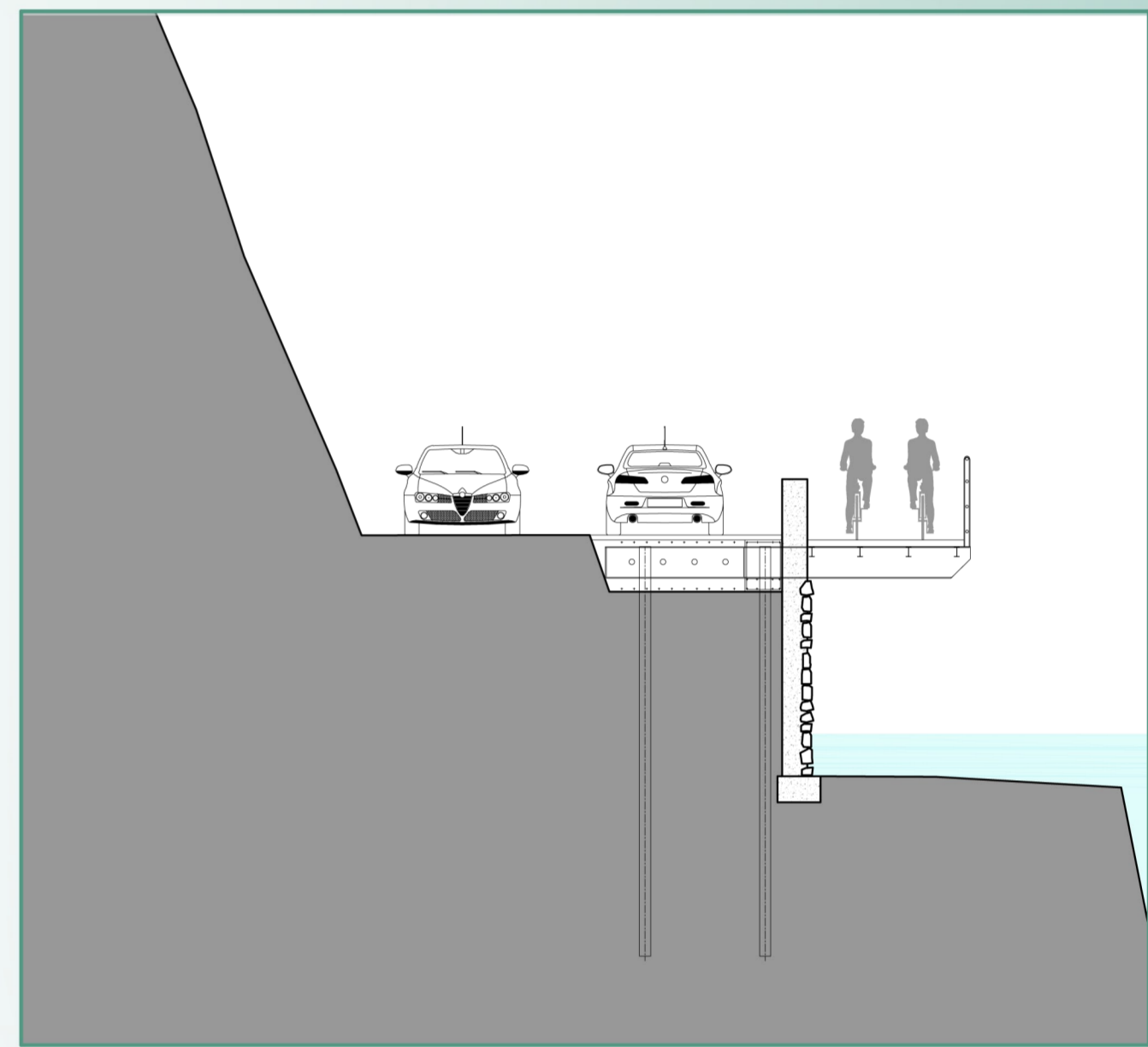
INSTALLAZIONE DI PASSERELLA A SBALZO ANCORATA ALLA STRADA
