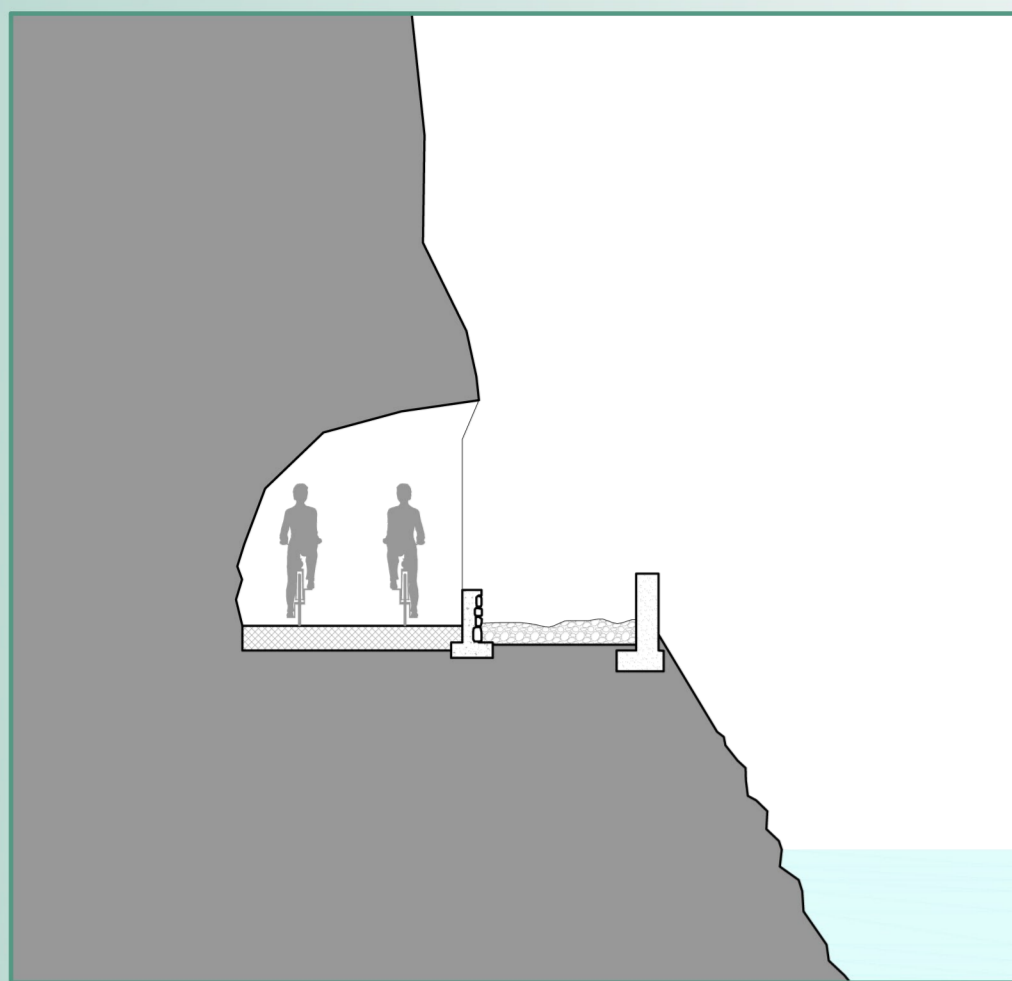
RIUSO DEL VECCHIO TRACCIATO CON SCAVO PARZIALE NELLA ROCCIA
