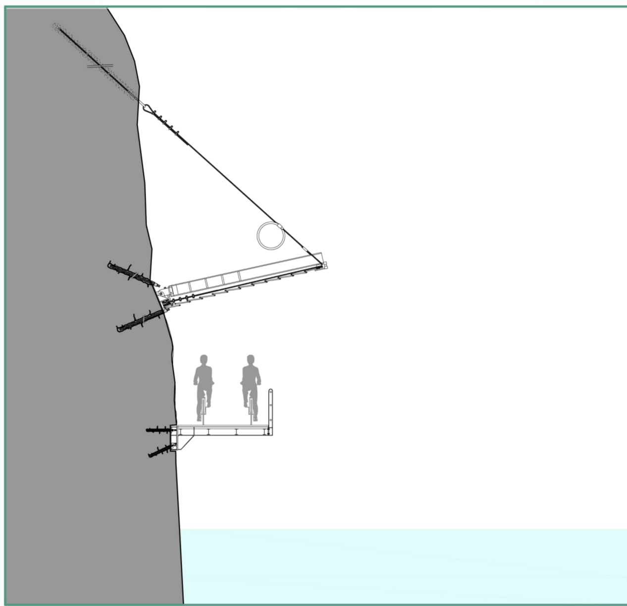
INSTALLAZIONE DI PASSERELLA A SBALZO ANCORATA ALLA ROCCIA
