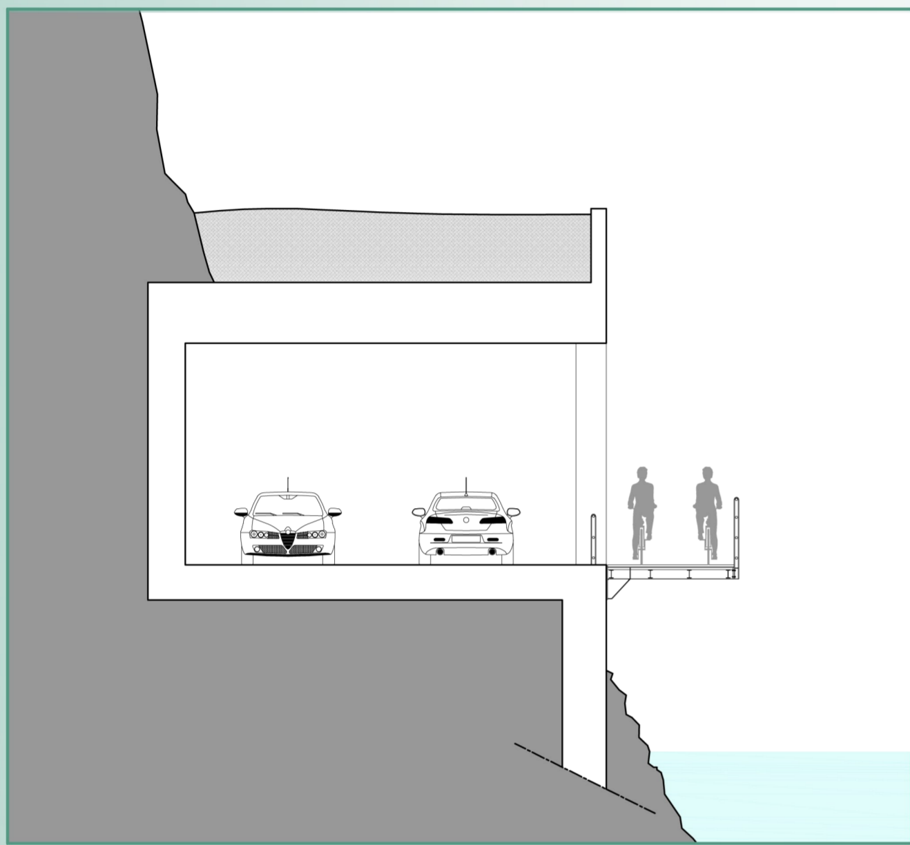
INSTALLAZIONE DI PASSERELLA A SBALZO ANCORATA ALLA GALLERIA PARAMASSI
