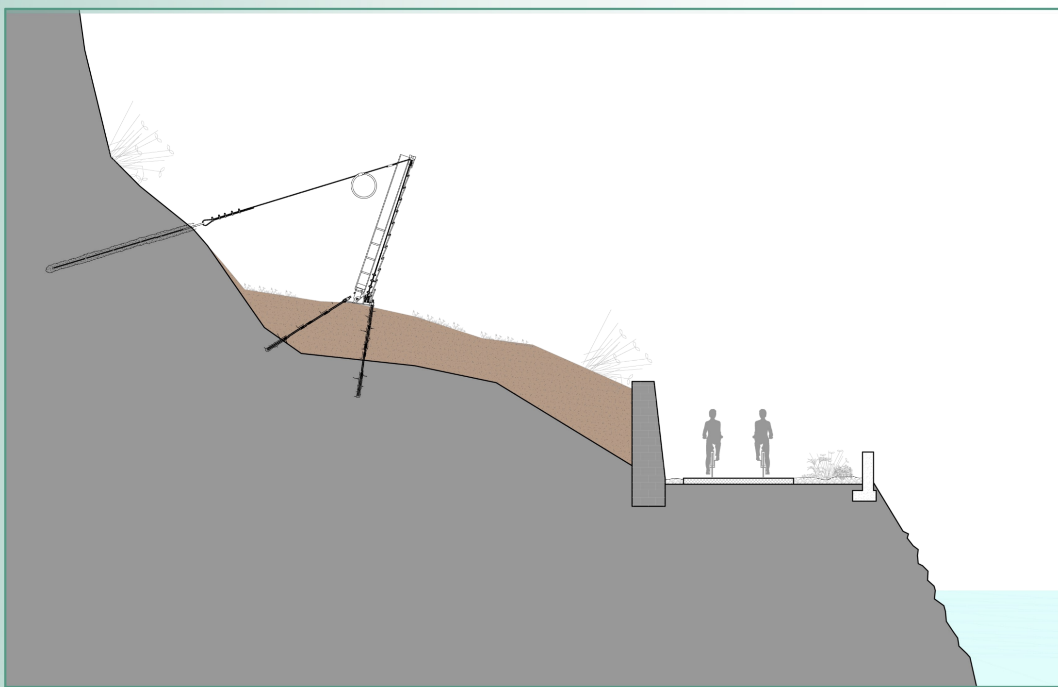
RIUSO DEL VECCHIO TRACCIATO CON SISTEMAZIONE DELLA PAVIMENTAZIONE
