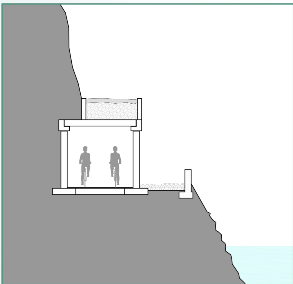
COSTRUZIONE DI NUOVA GALLERIA ARTIFICIALE CON SCAVO PARZIALE NELLA ROCCIA
