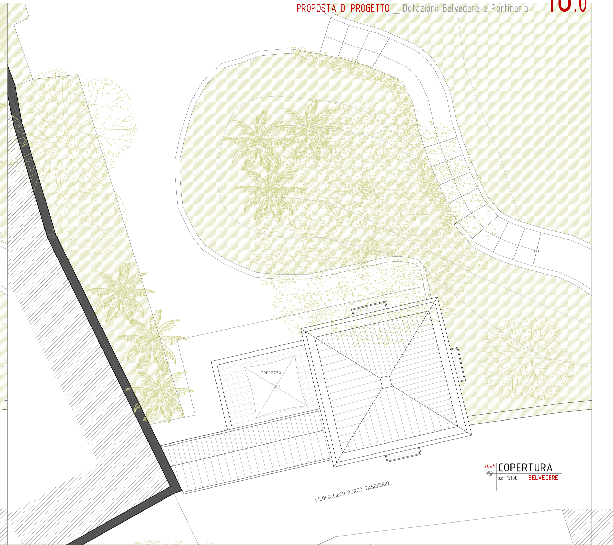
+445 PIANO PRIMO sc. 1:100 BELVEDERE
