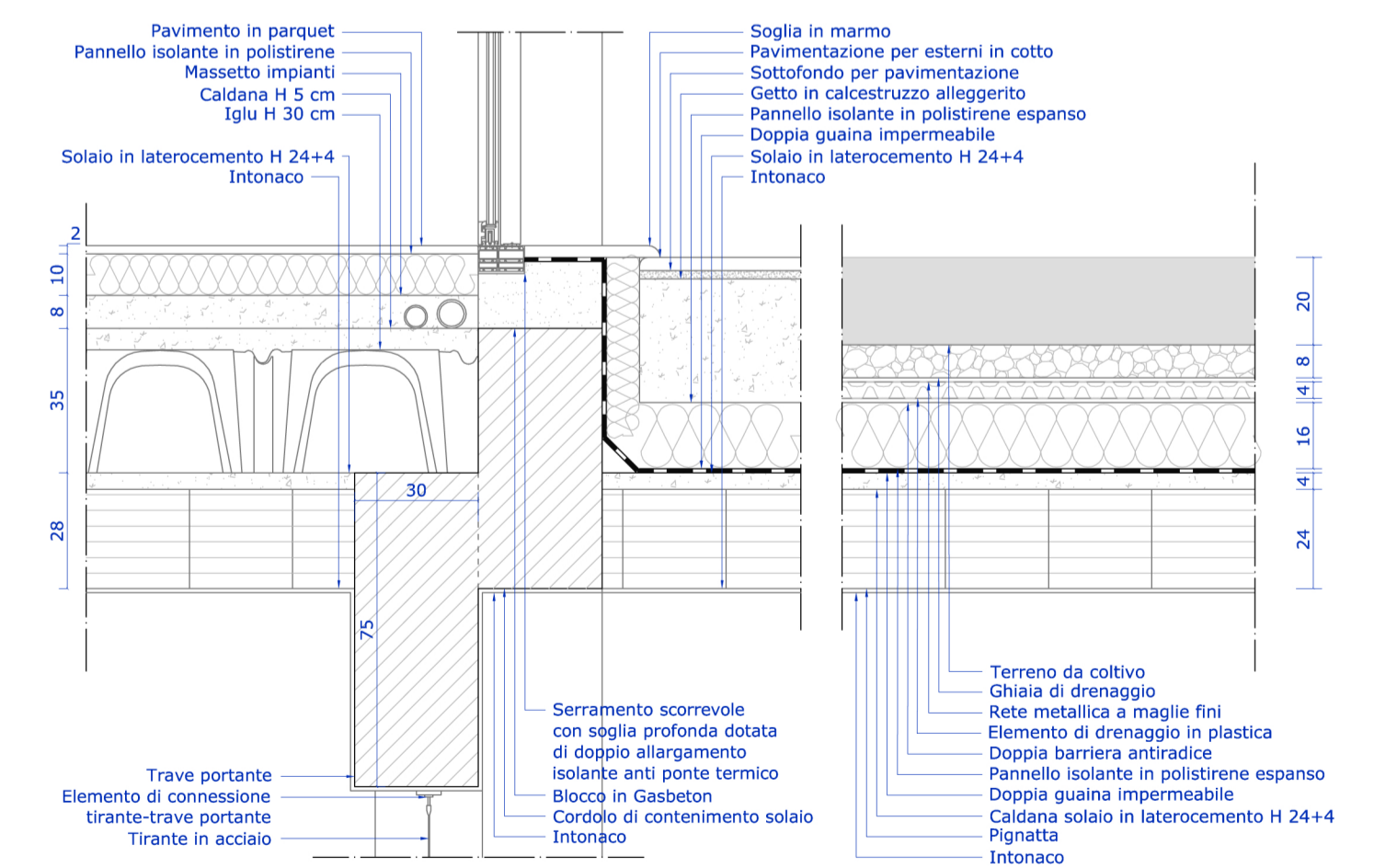
DETTAGLIO SOLAIO INTERNO/SOLAIO ESTERNO _SCALA 1:20
