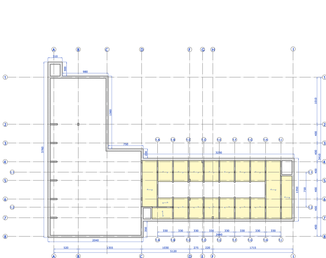
TERZO PIANO INTERRATO
