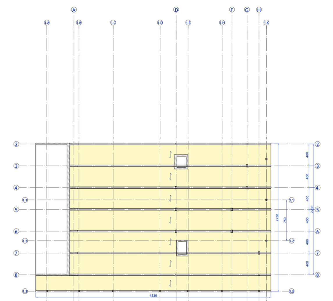
PRIMO PIANO FUORI TERRA
