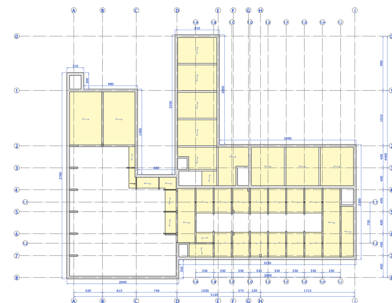
SECONDO PIANO INTERRATO
