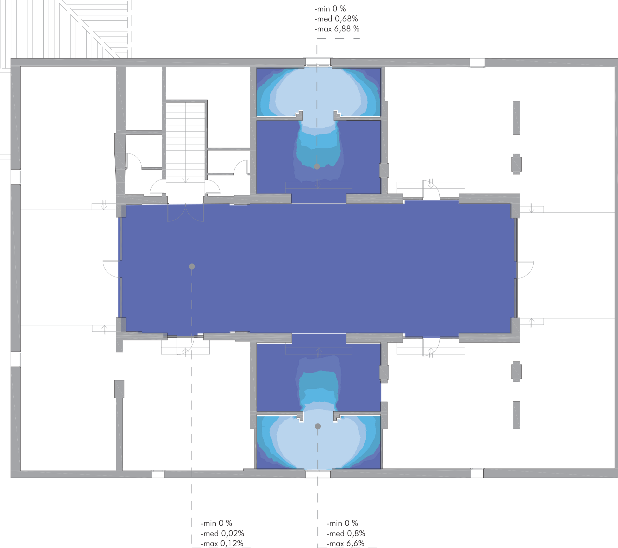
CALCOLO DELLA LUMINANZA
