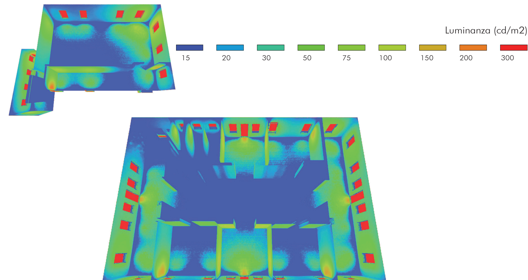
CALCOLO DELLA LUMINANZA
