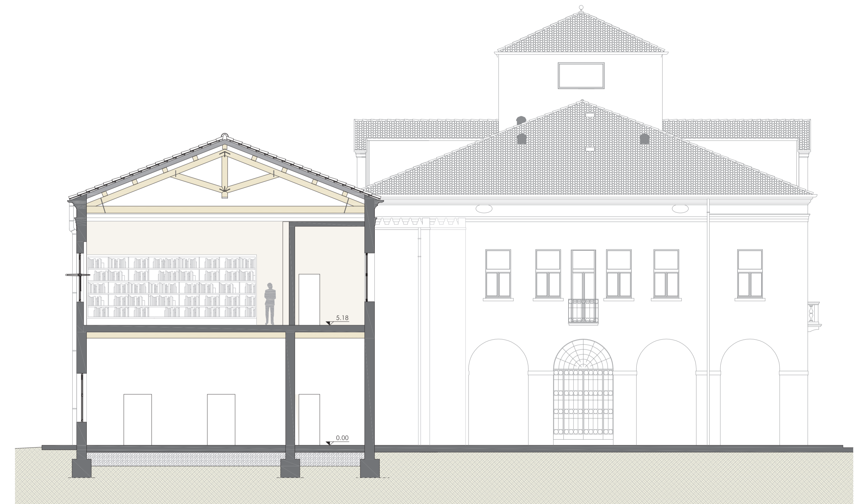
SEZIONE DD
