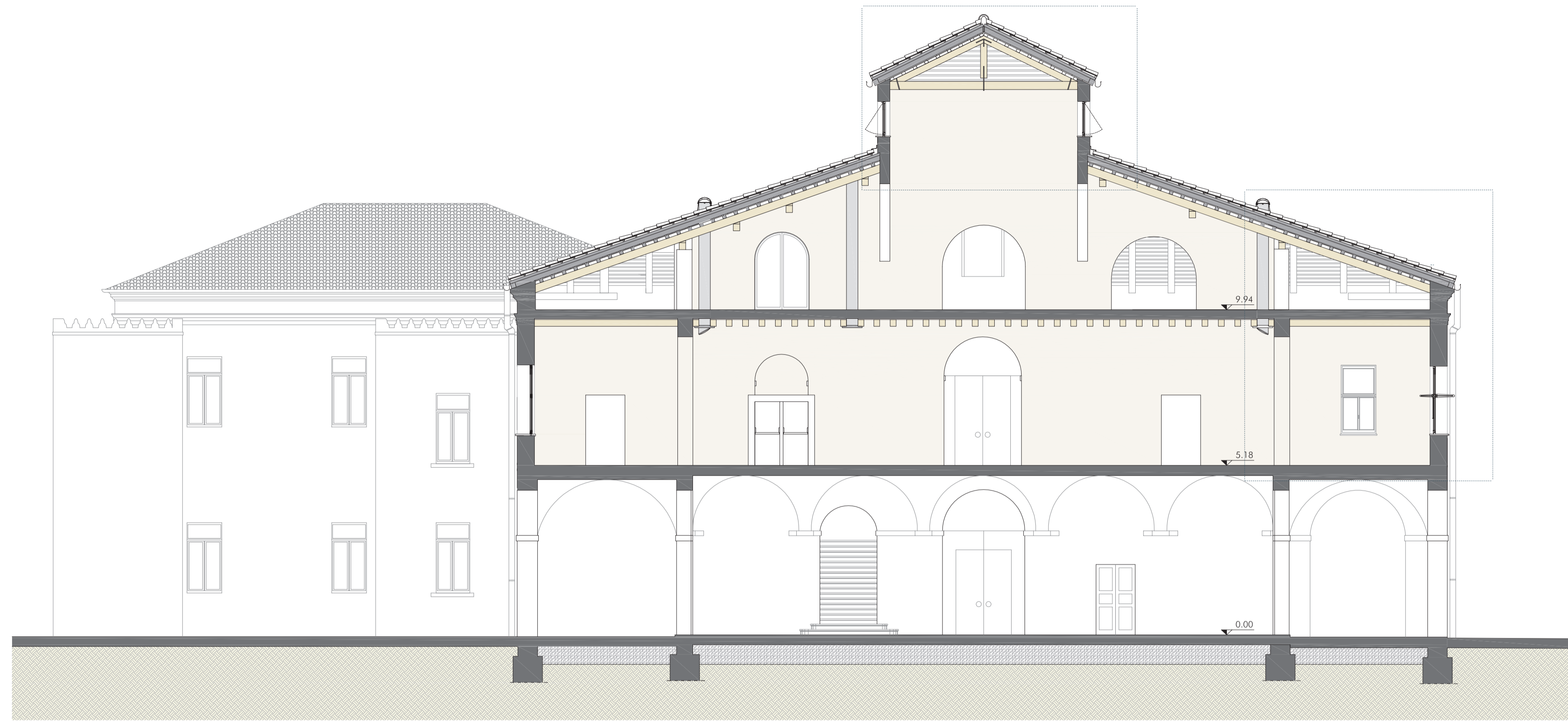
SEZIONE AA
