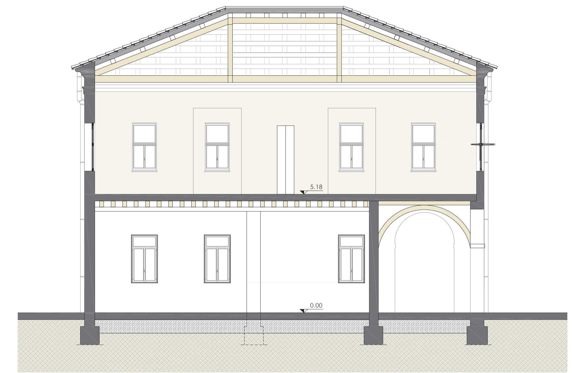
SEZIONE CC
