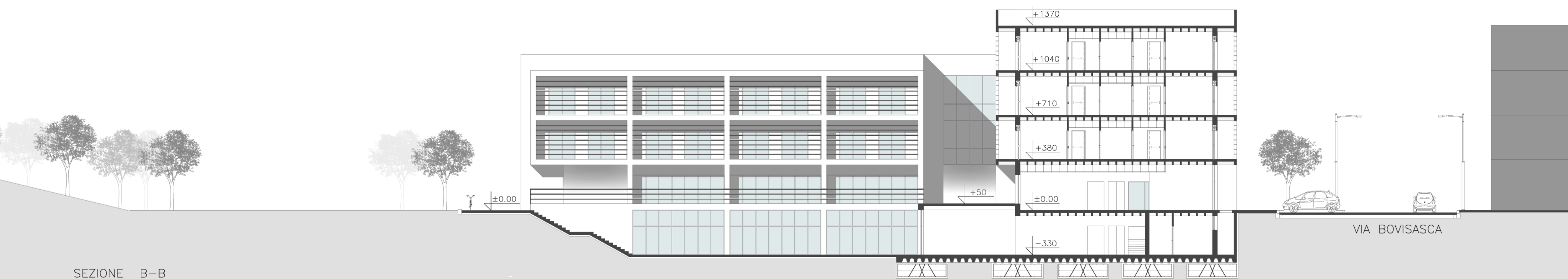
SEZIONE B-B
