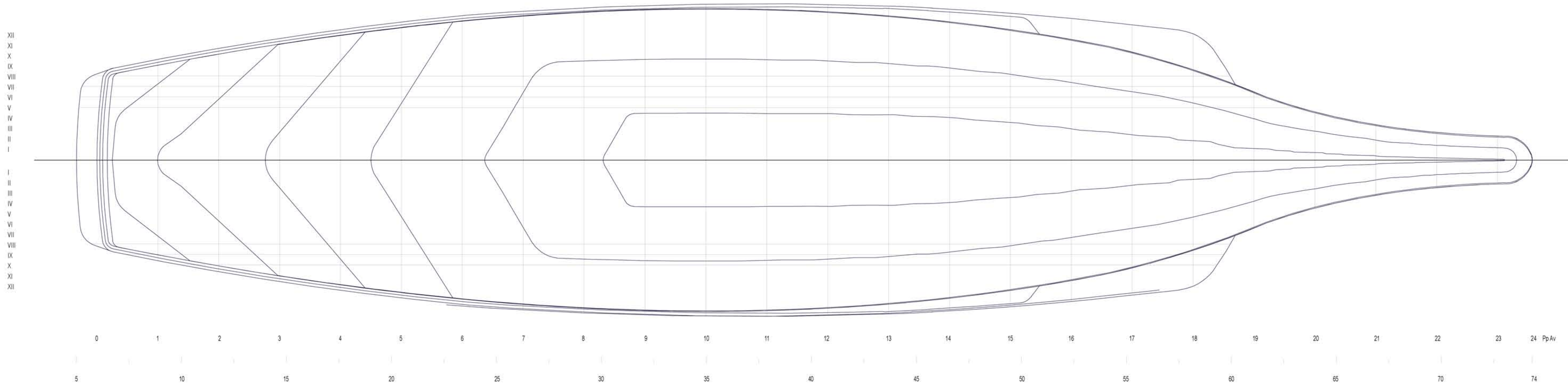
Piano delle Linee d'acqua _Pianta
