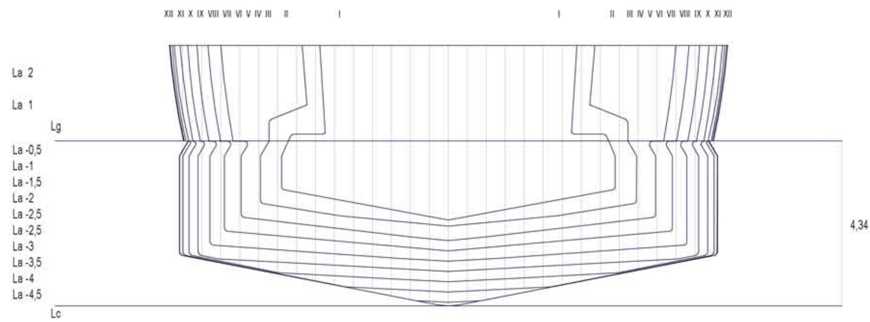
Piano delle Ordinate _Sezioni verticali Poppa
