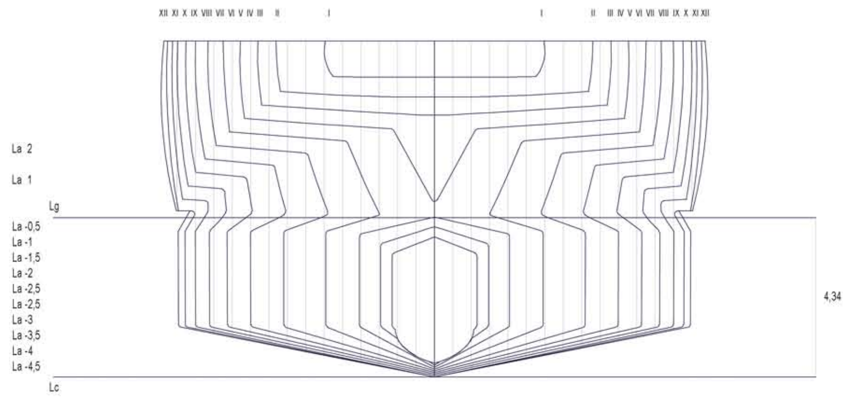
Piano delle Ordinate _Sezioni verticali Prua
