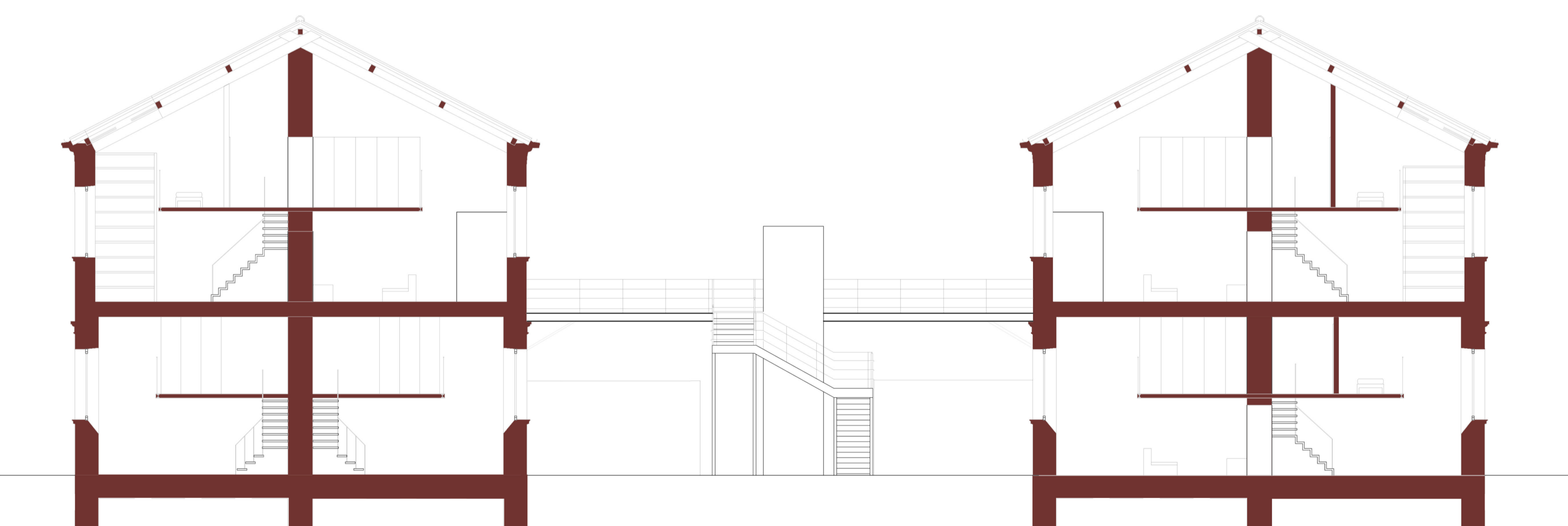
SEZIONE AA
