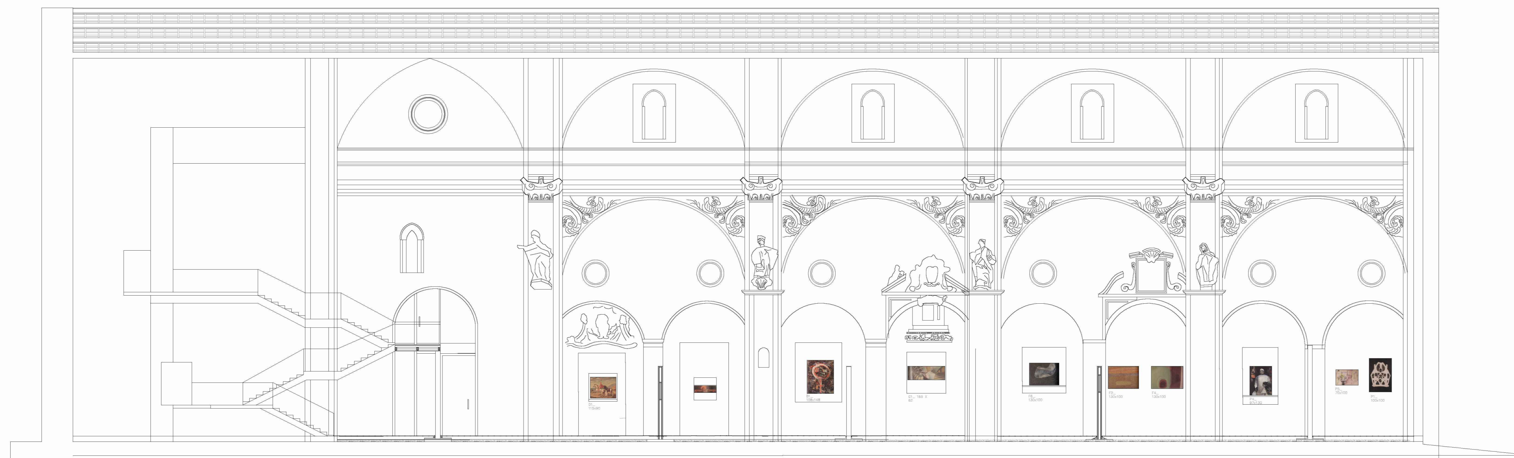
Rilievo geometrico scala 1:50
