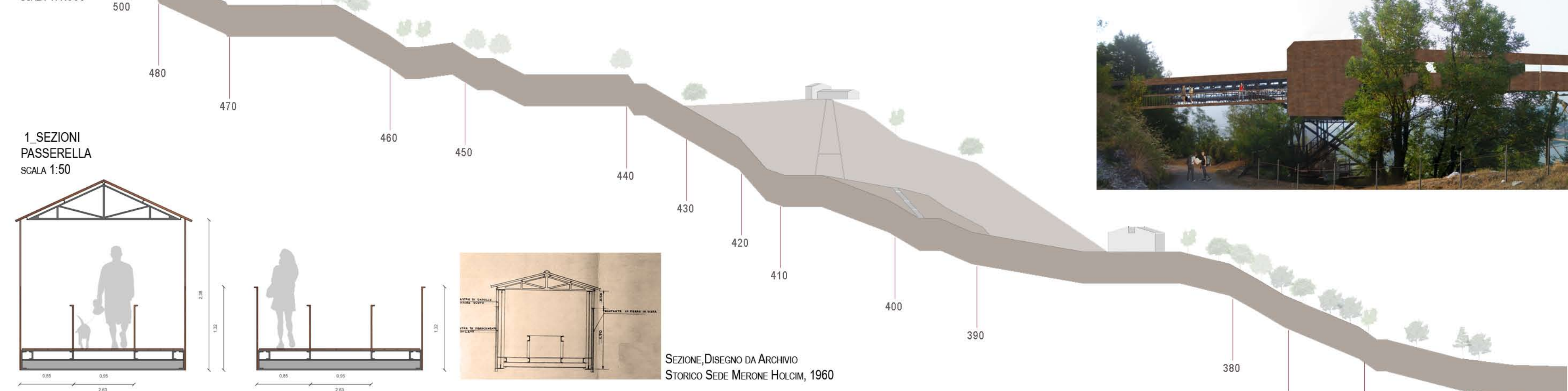
SEZIONE TERRITORIALE 2 SCALA 1:1.000
