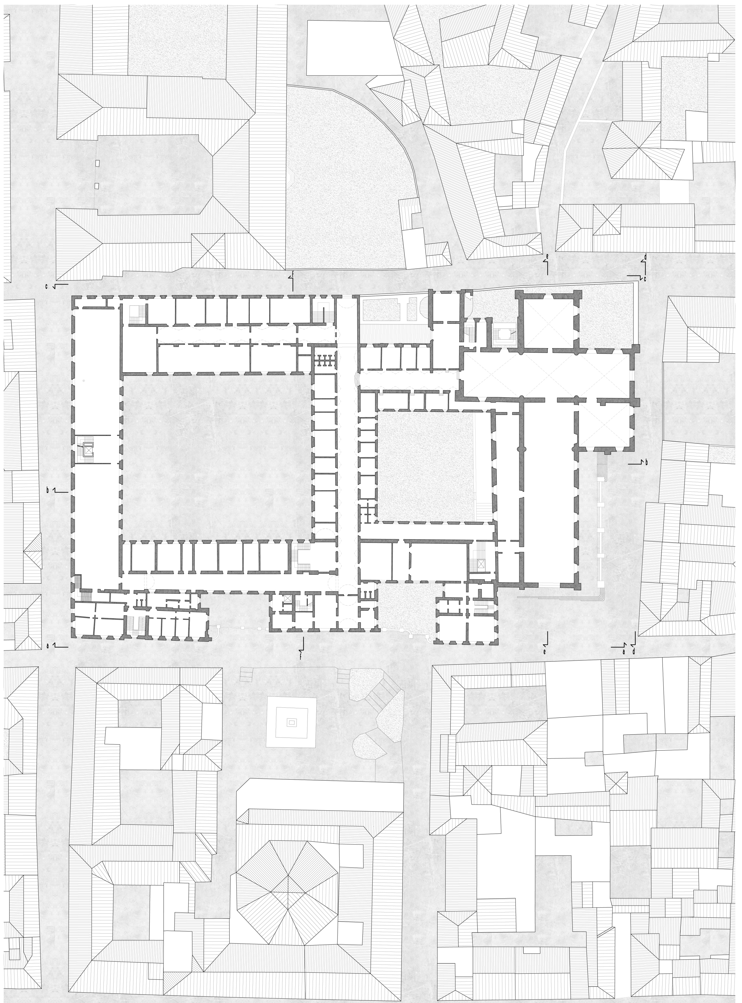
STATO DI FATTO - Piano piano primo 1500
