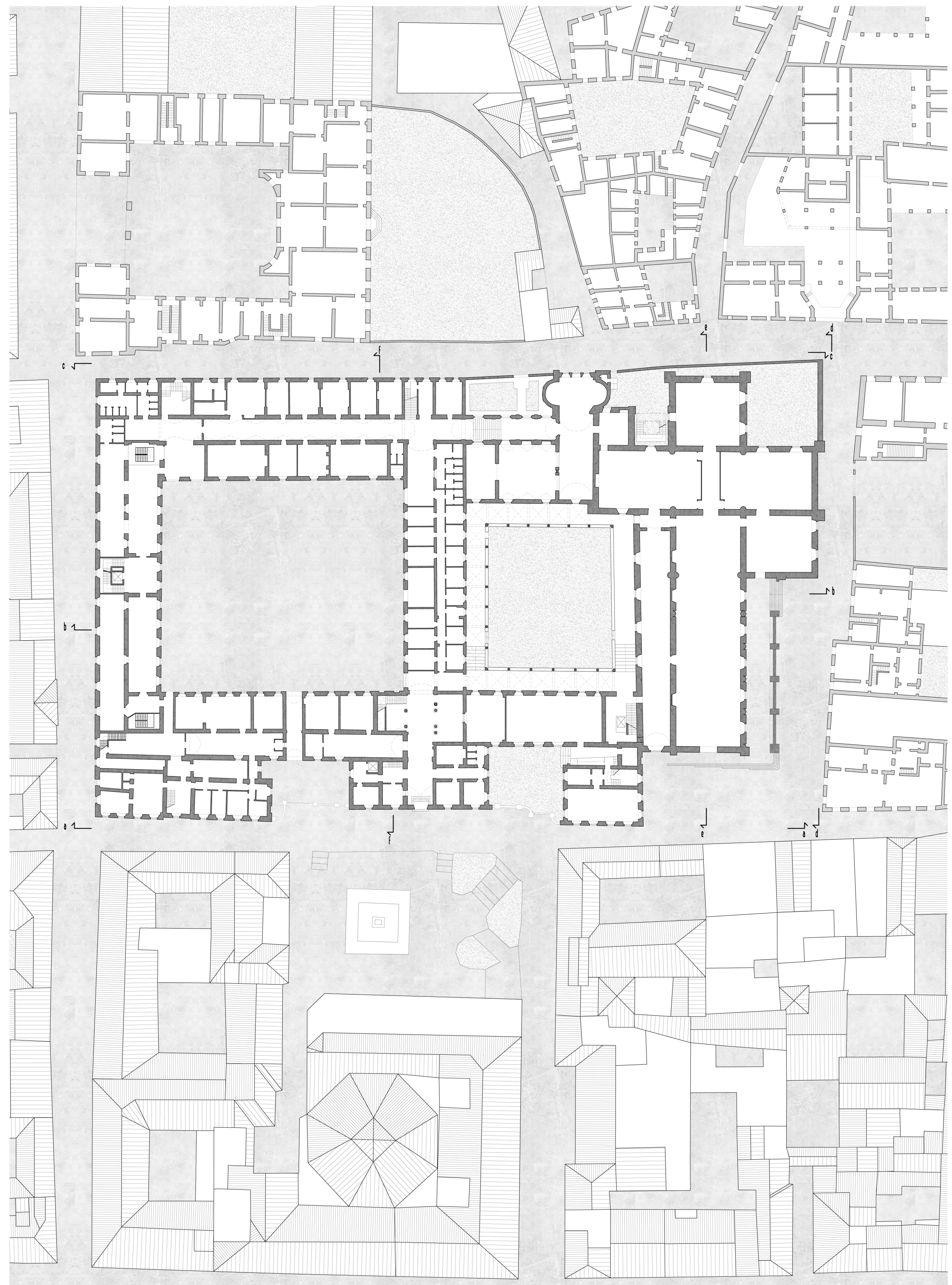
STATO DI FATTO - Piano piano terra 1500
