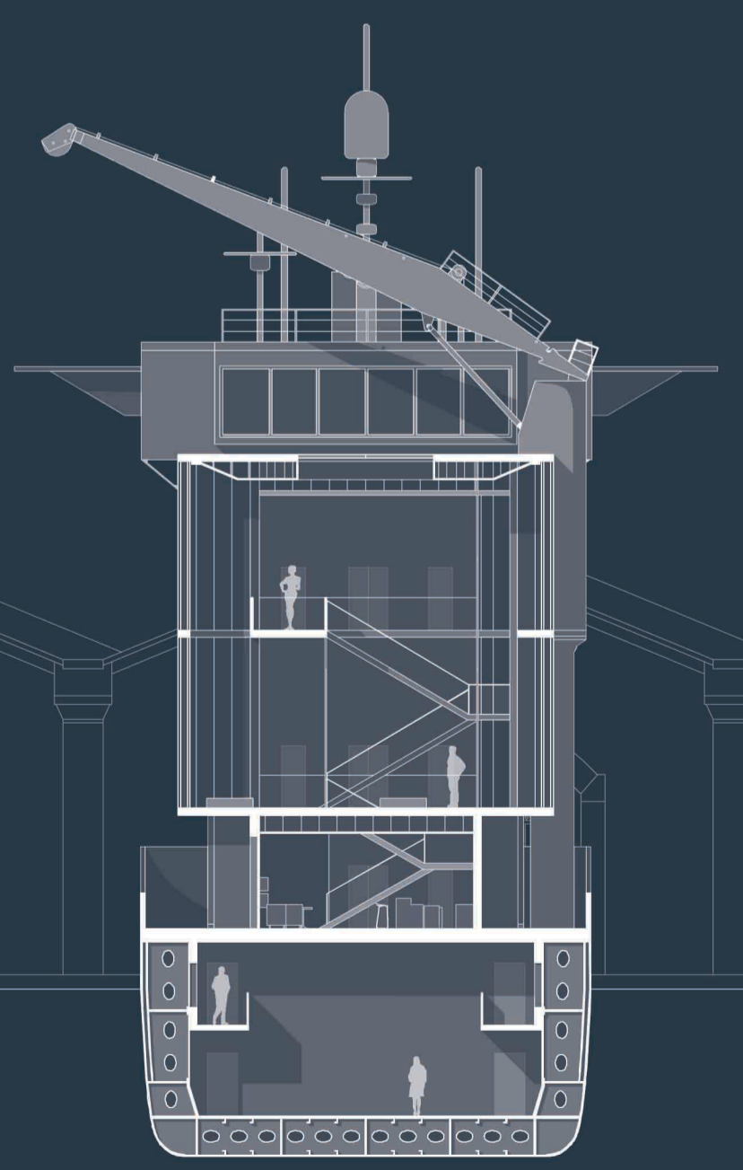
SEZIONE DD
