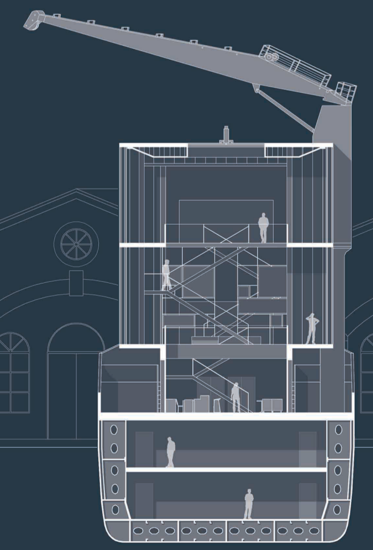
SEZIONE CC
