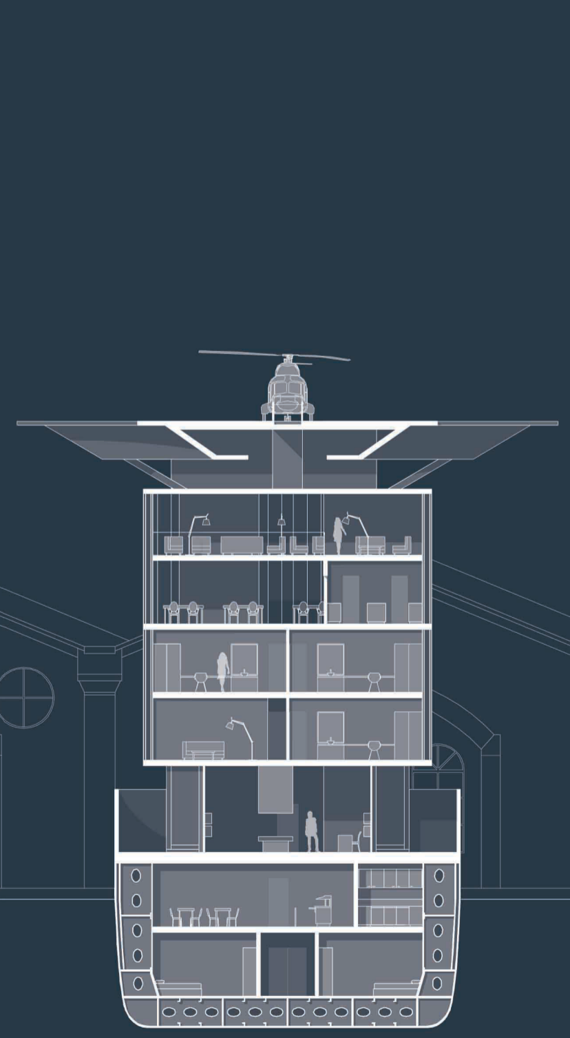
SEZIONE BB
