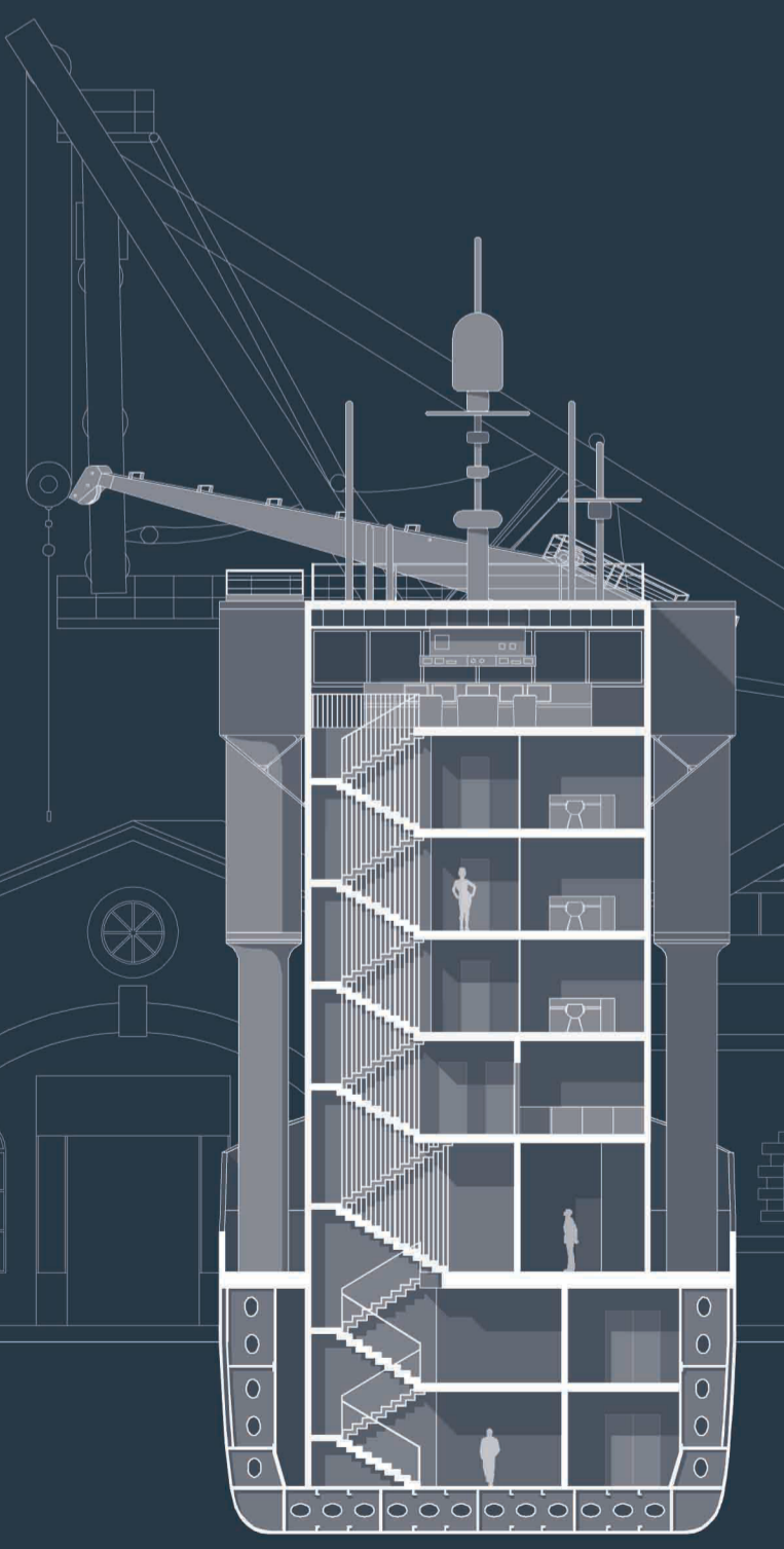
SEZIONE EE
