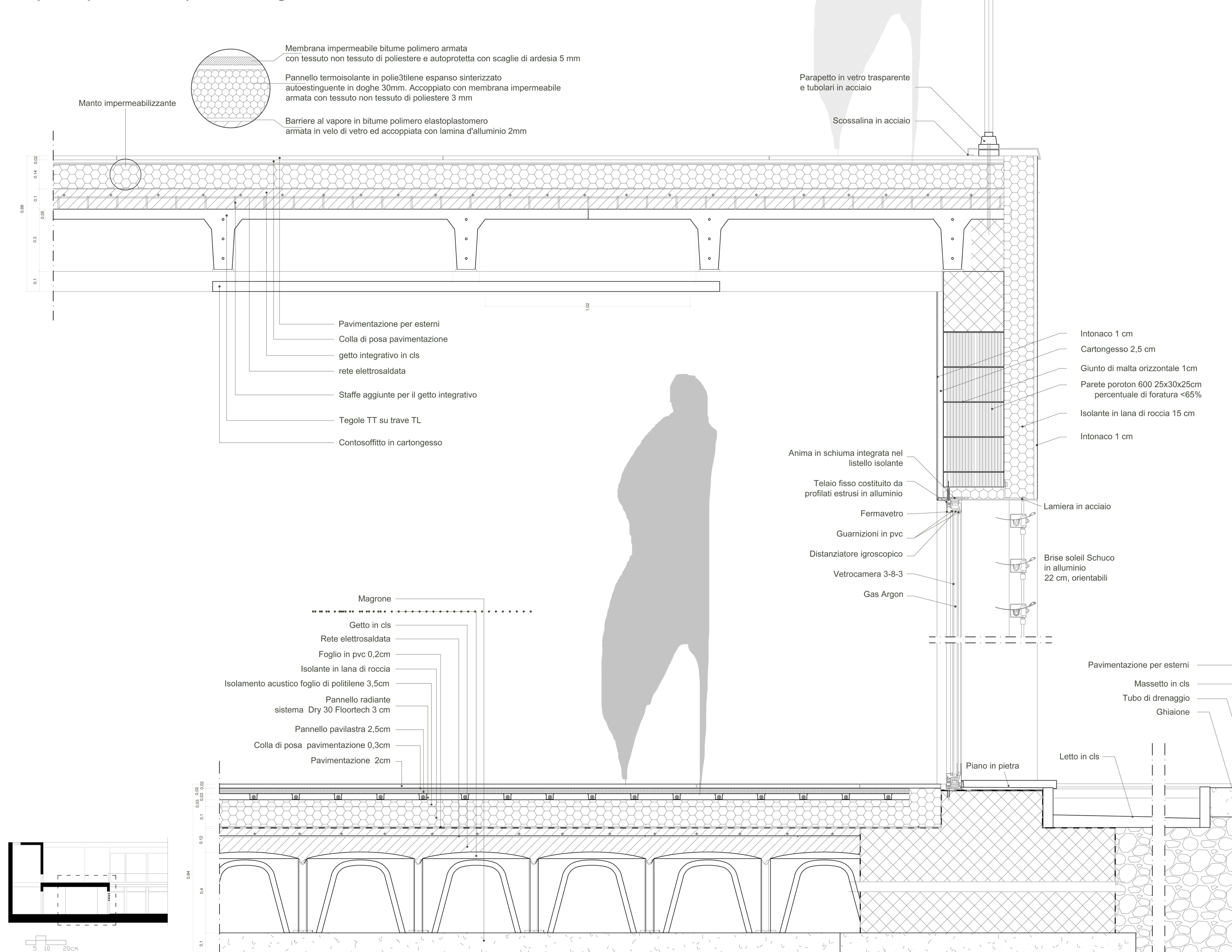
SEZIONE STRUTTURALE MUSEO: Copertura praticabile con pendenza ortogonale alla sezione.
