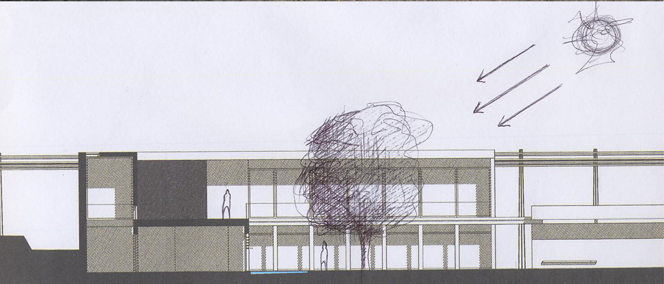
SEZIONE STRUTTURALE MUSEO: Copertura praticabile con pendenza ortogonale alla sezione.
