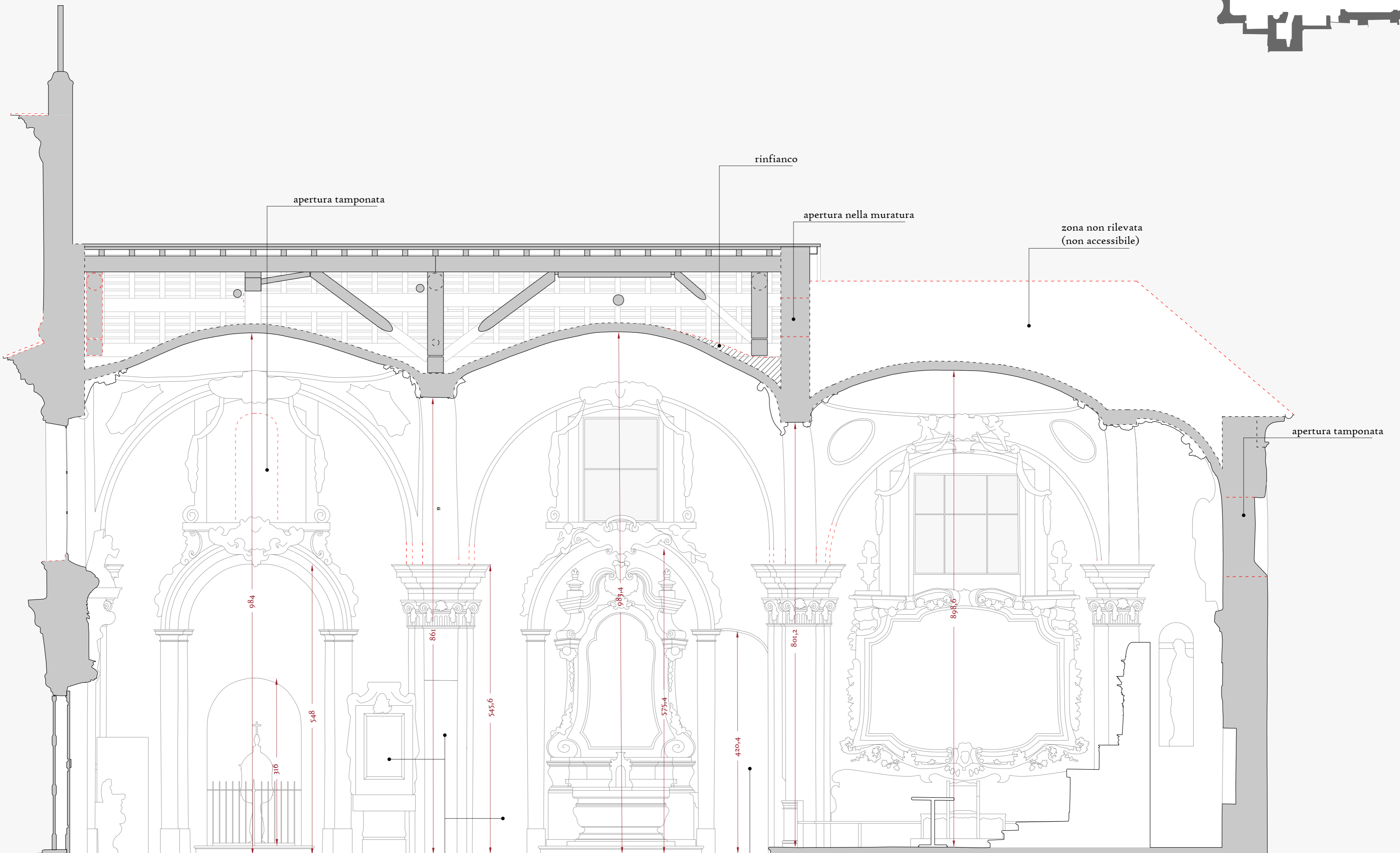
rilievo geometrico
