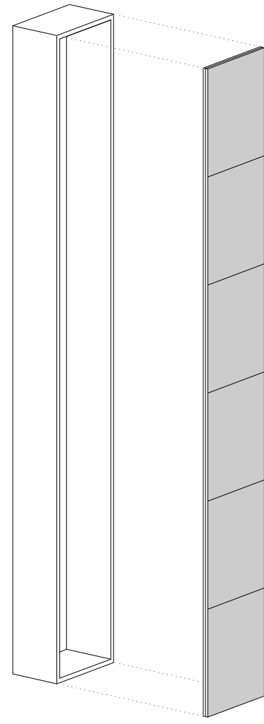
CELLULA SEMI-TRASPARENTE VETRO FOTOVOLTAICO DOPPIA CAMERA M Clear (10% Trasparenza) CELLULA 60x360m
