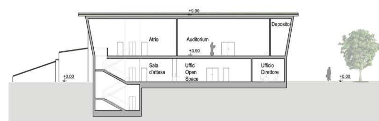
Sezione C-C'
