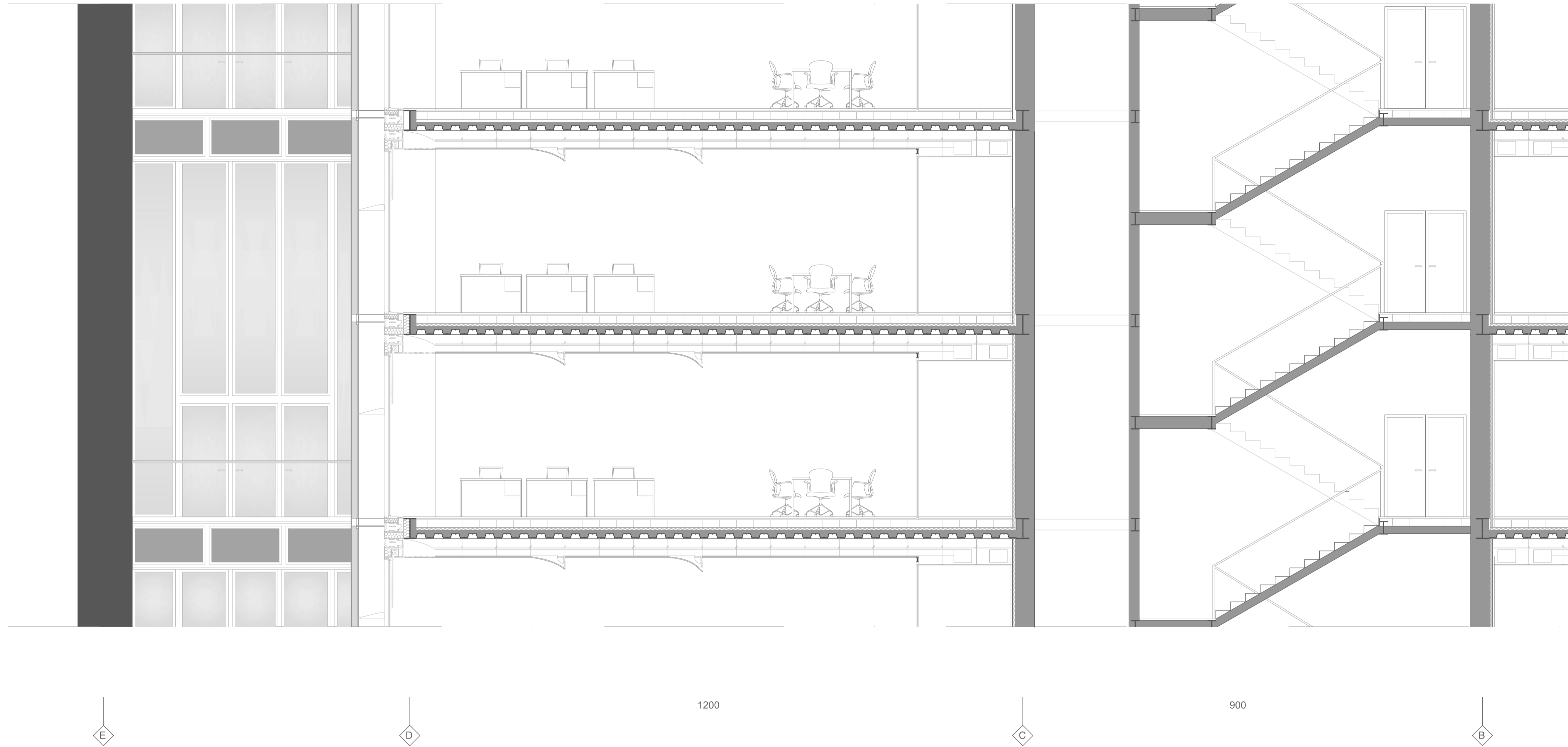
SEZIONE A-A 1:50
