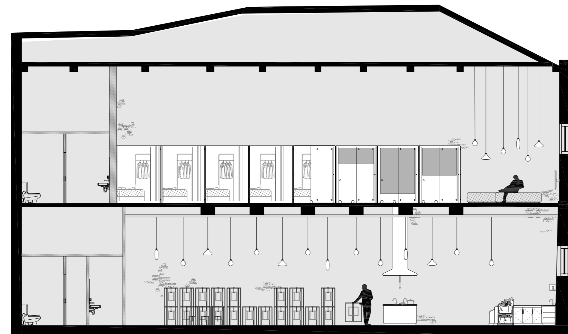
SEZ D-D'
