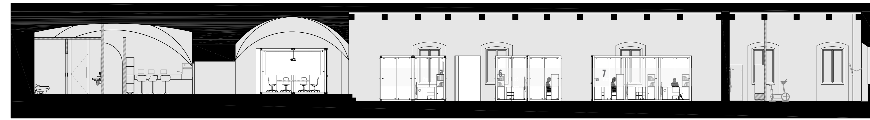
SEZ F-F'
