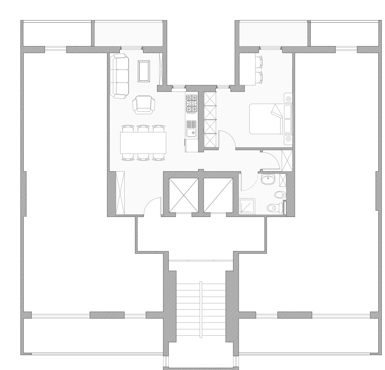
48 mq
