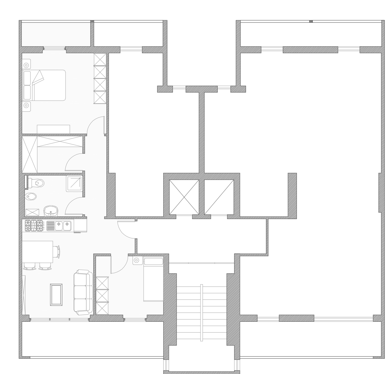
50 mq
