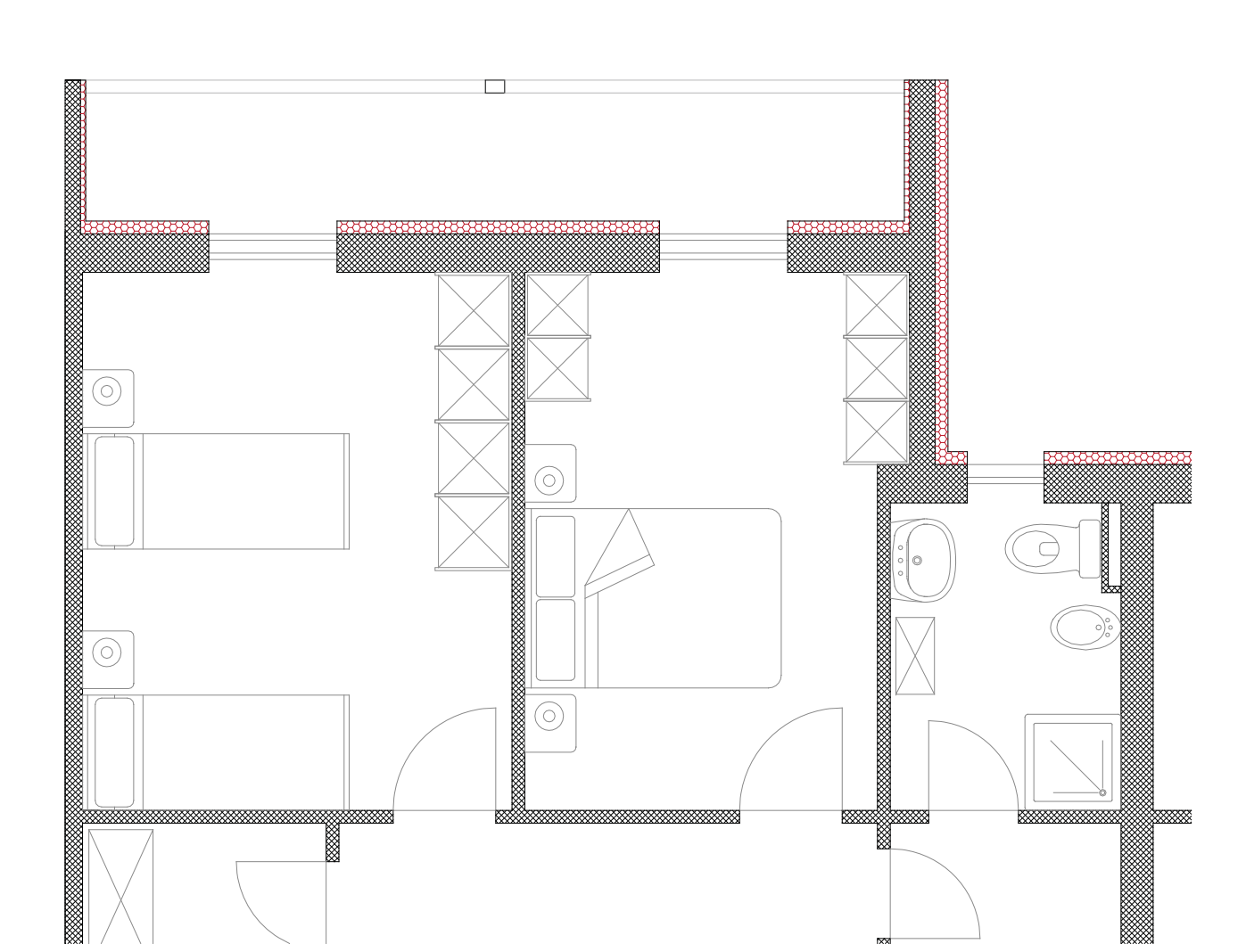
CORREZIONE PONTE TERMICO
