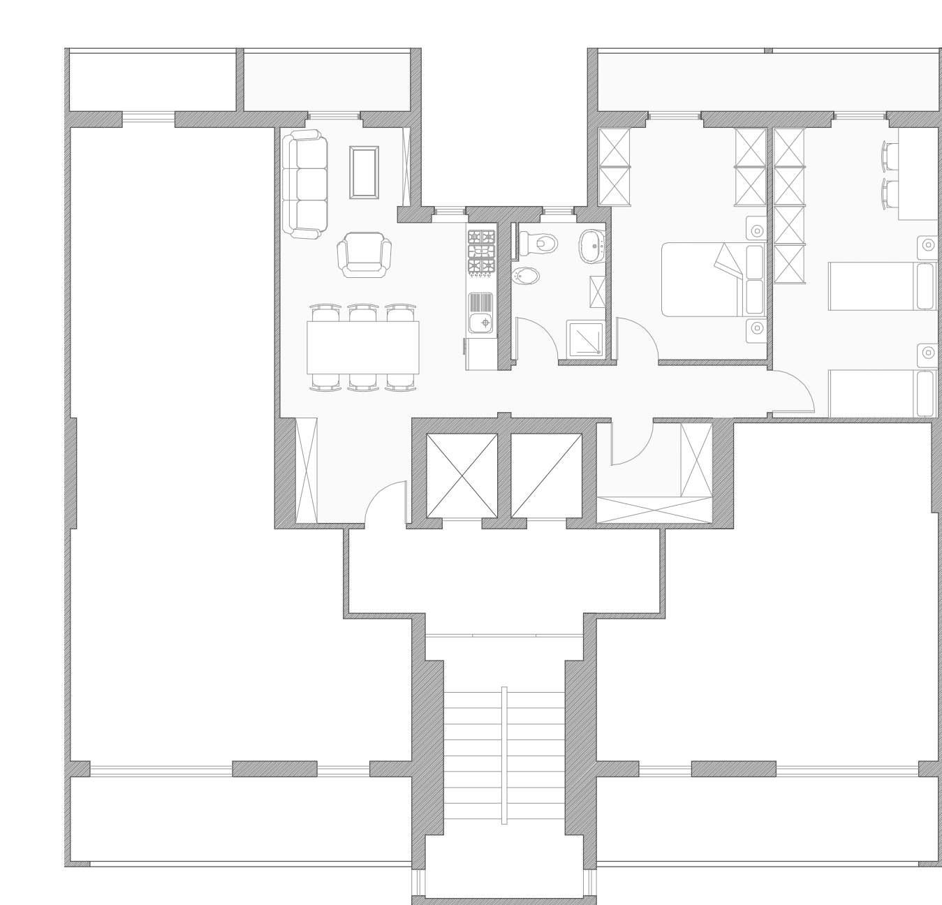
65 mq
