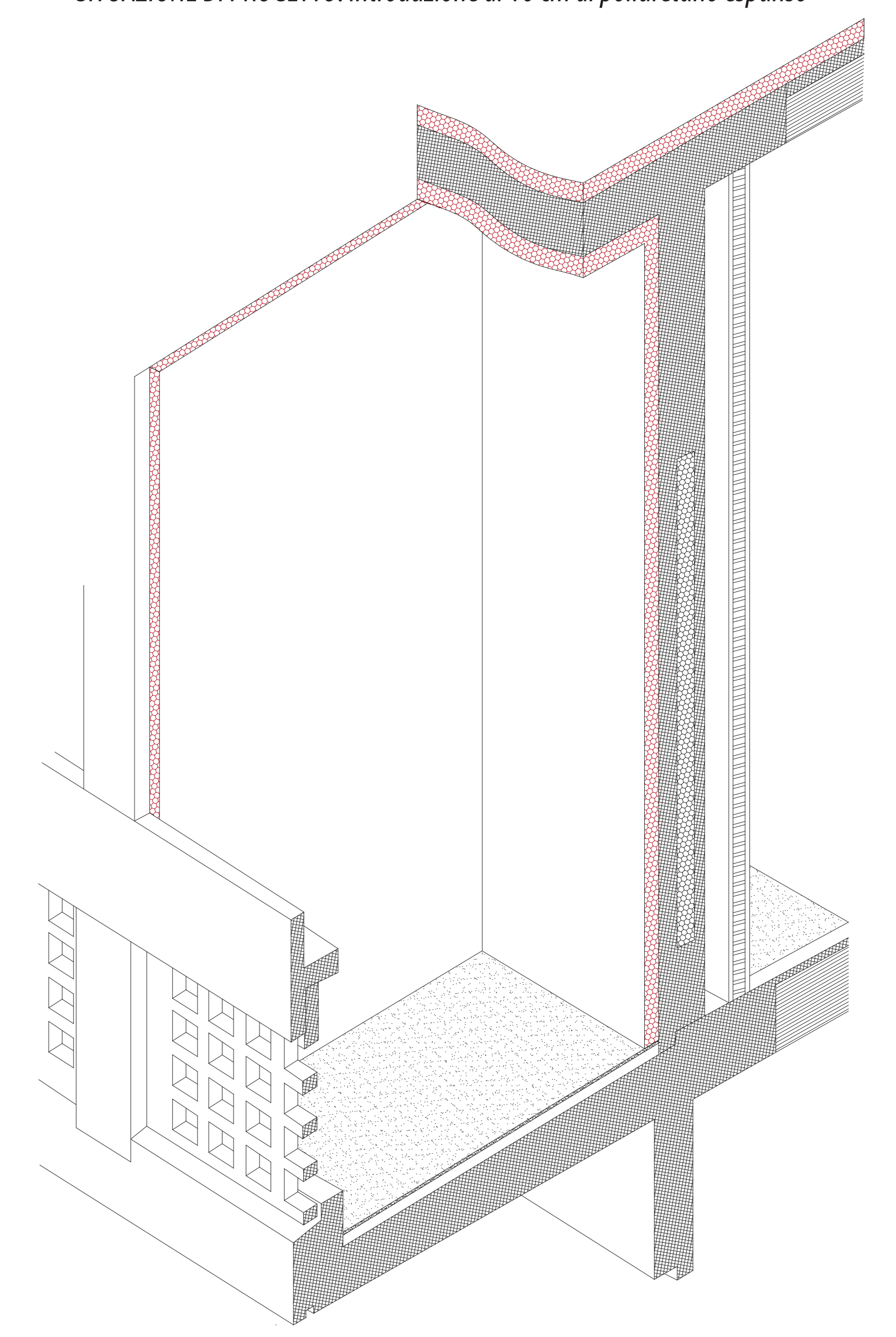
CORREZIONE PONTE TERMICO
