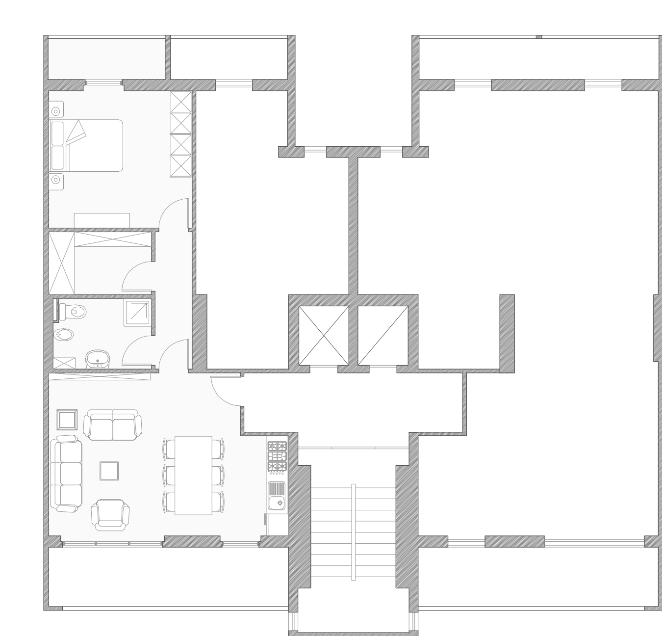
50 mq
