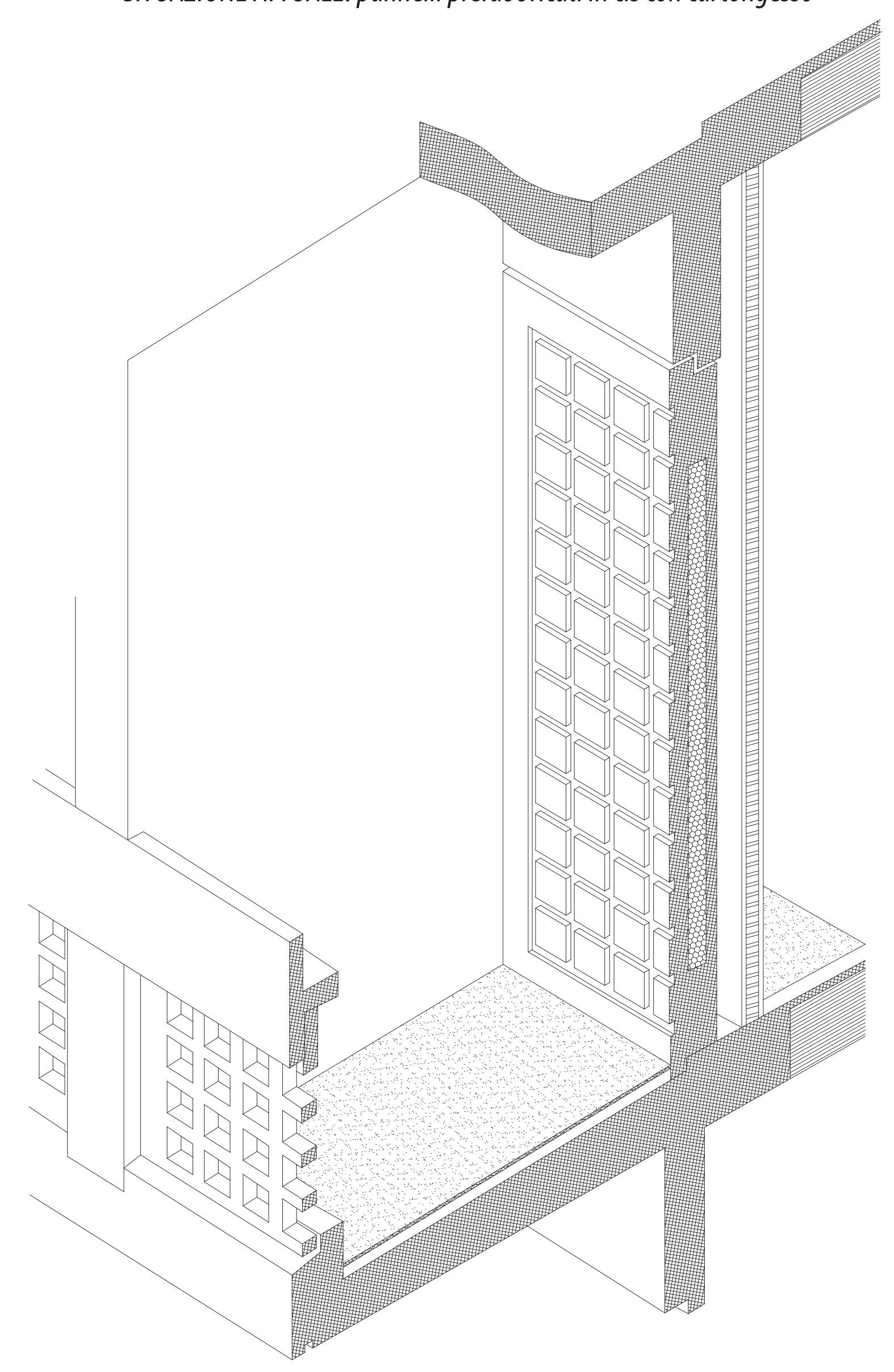
SCHEMA PASSAGGIO IMPIANTI
