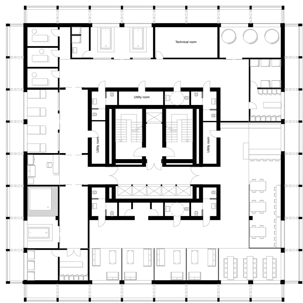
PIANTA ULTIMO PIANO 1:200
