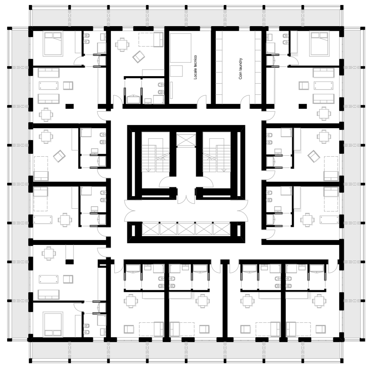
PIANTAPIANO TIPO RESIDENZA 1:200
