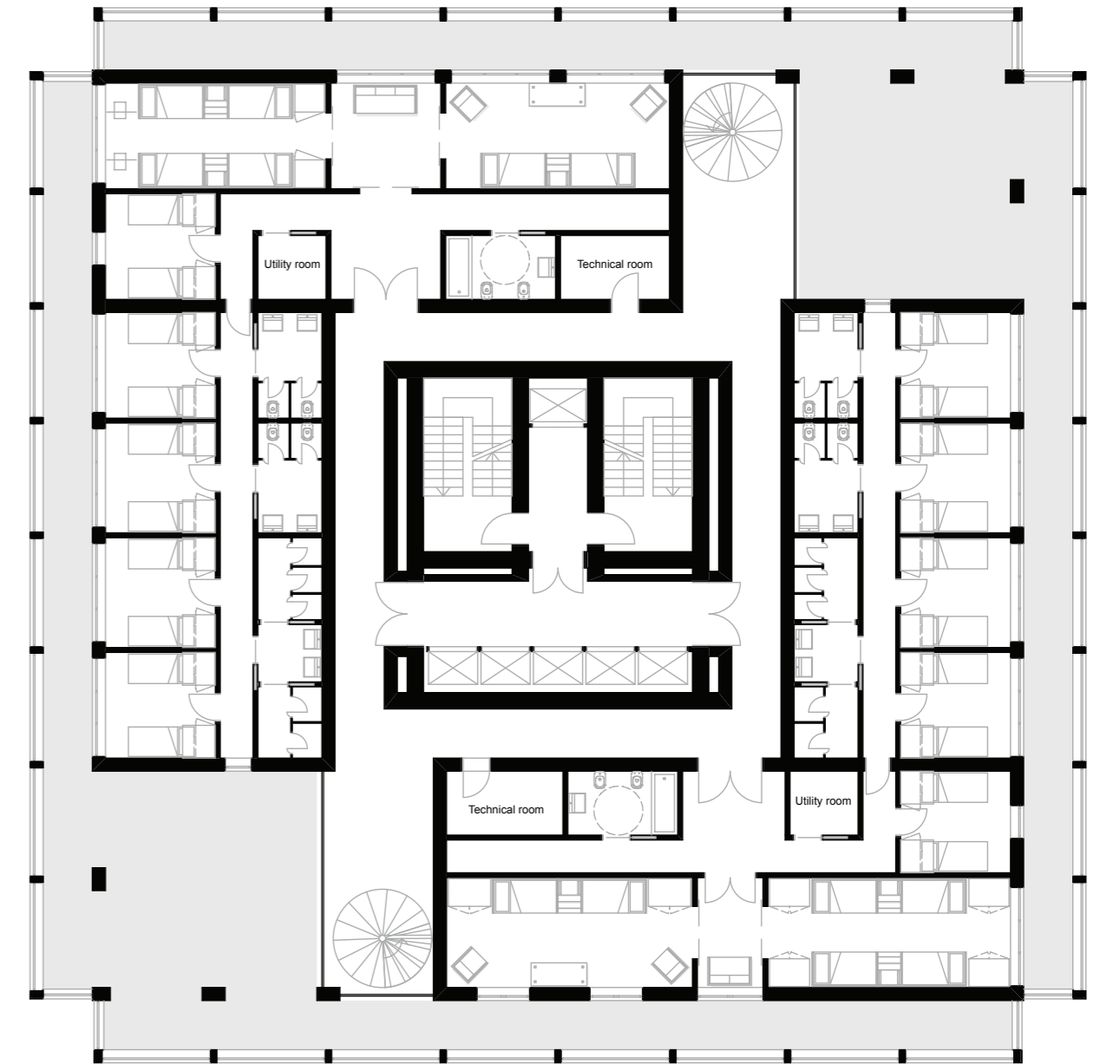
PIANTE BLOCCO OSTELLO TIPO 1
