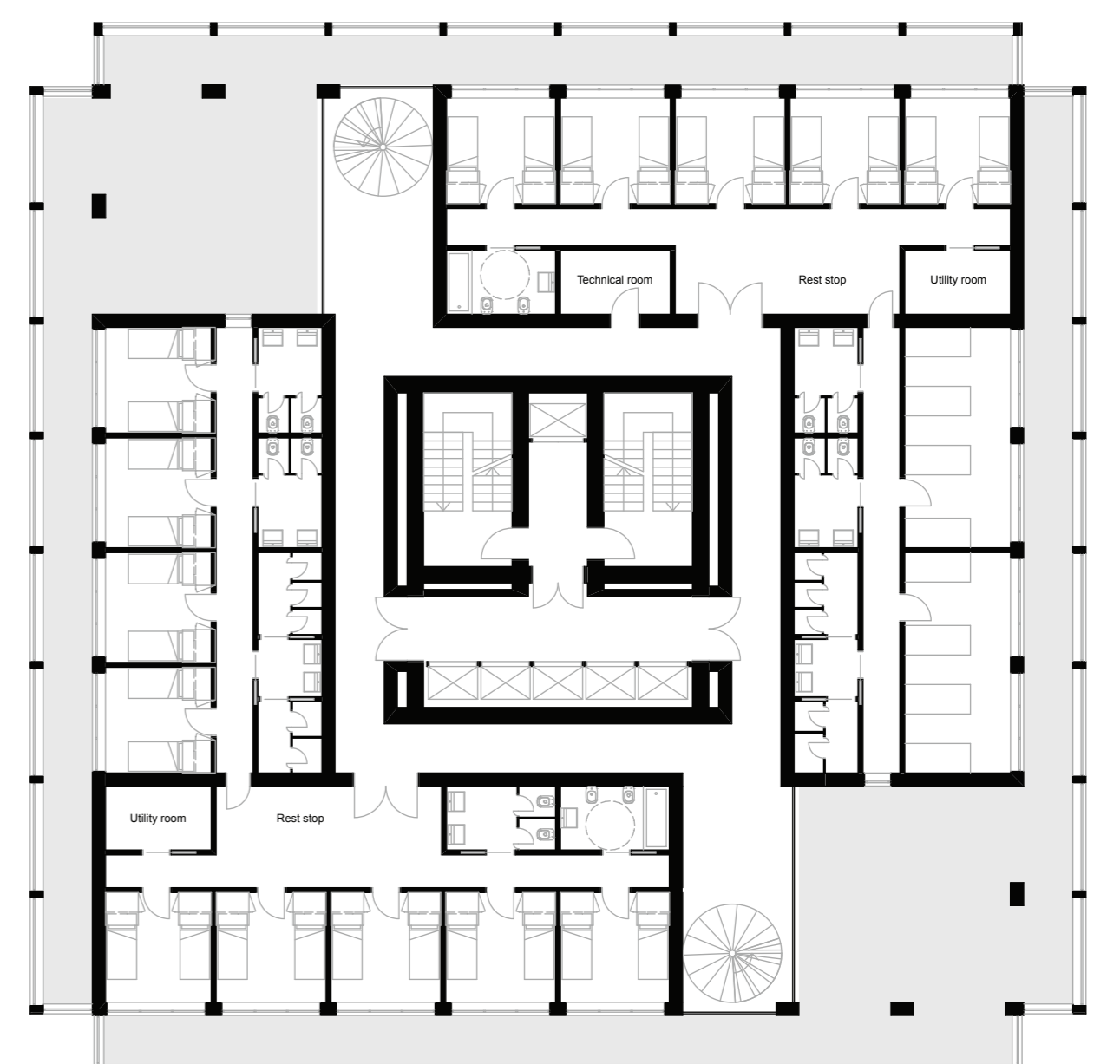
PIANTE BLOCCO OSTELLO TIPO 2
