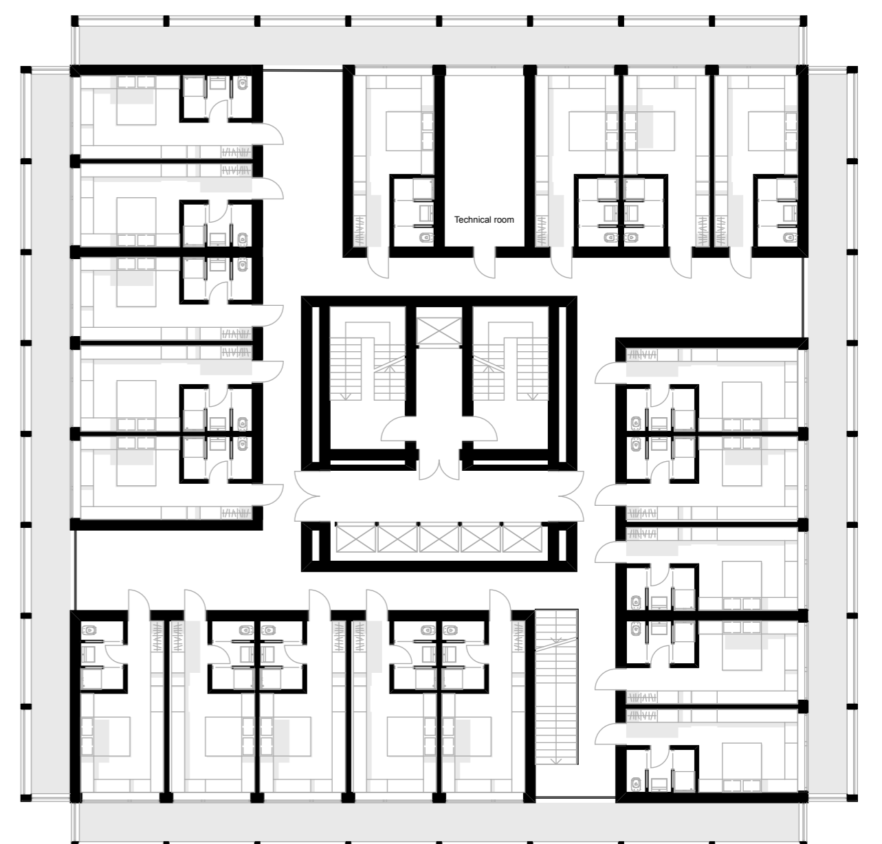
PIANTE BLOCCO TIPO HOTEL 1:200
